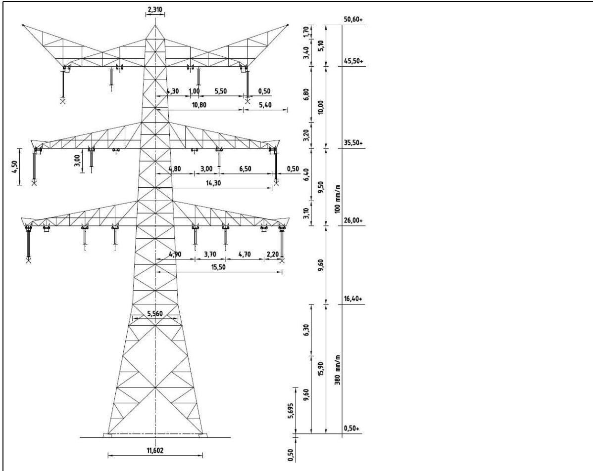
Figuur 2 Mastbeeld masttype EA-3/co
