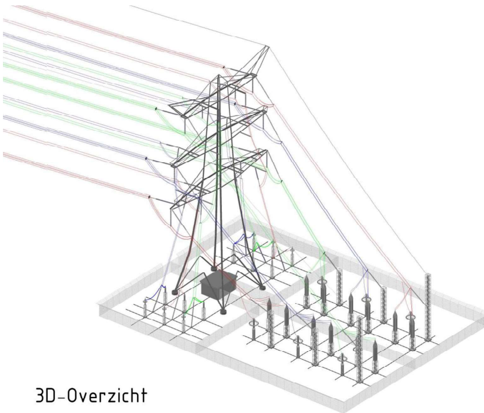
Figuur 1 Principeontwerp EA-3/co-eindmast
