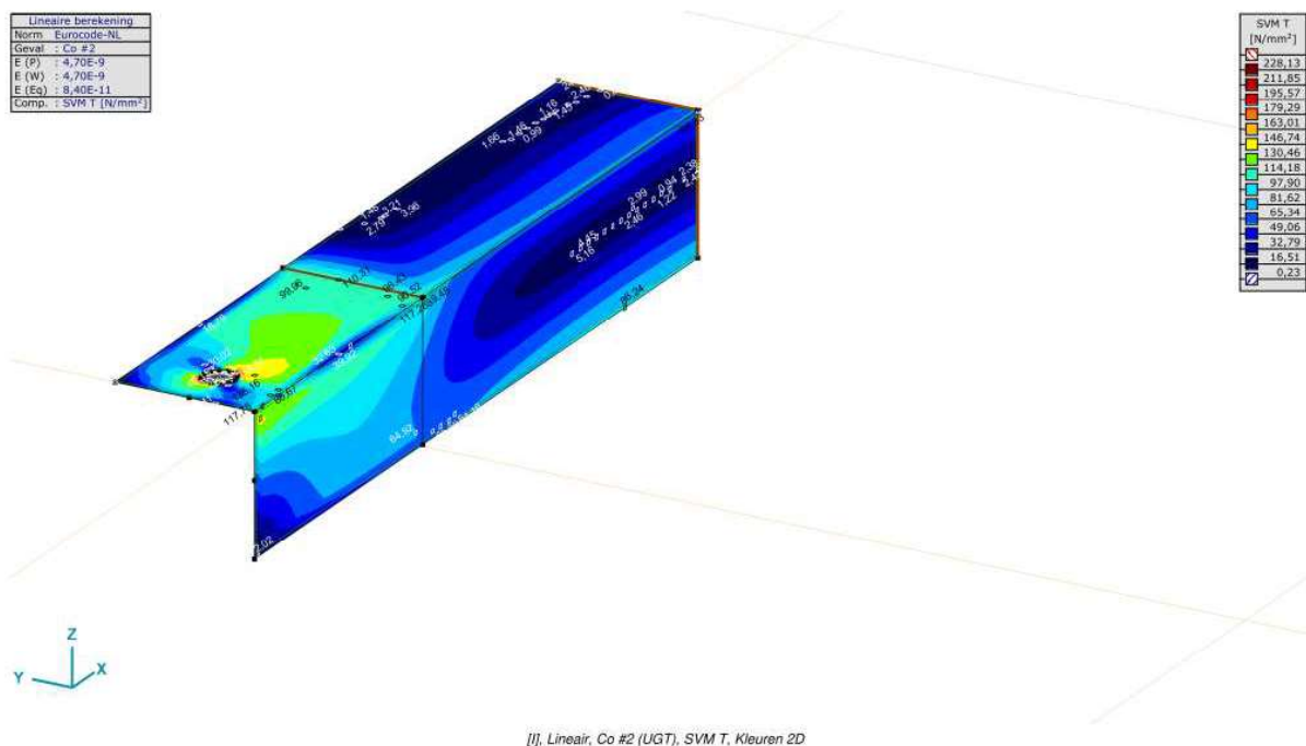
Figuur 3 Maximale spanning in hoekprofiel voor 380 kV
