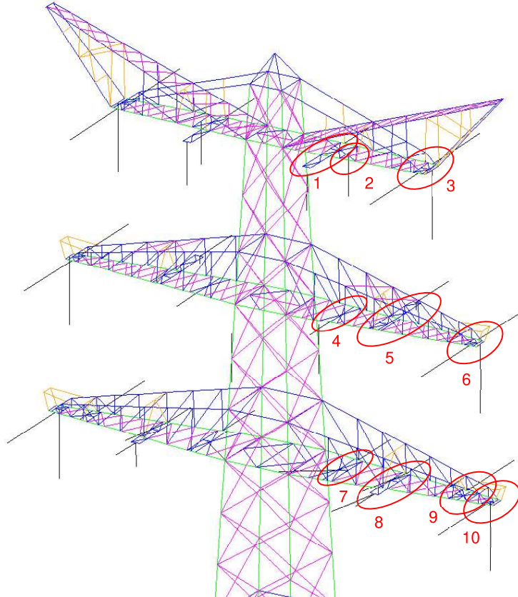
Figuur 1 Overzicht van liggers
