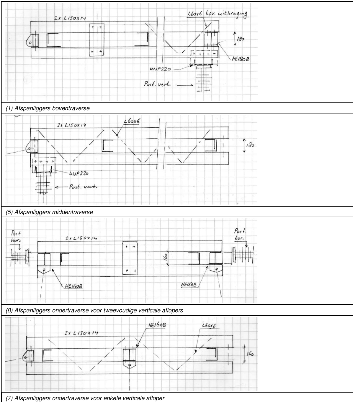
Figuur 2 Principe afspanliggers
