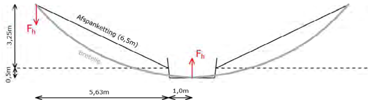
Figuur 2 Boveanzaicht bretelle
