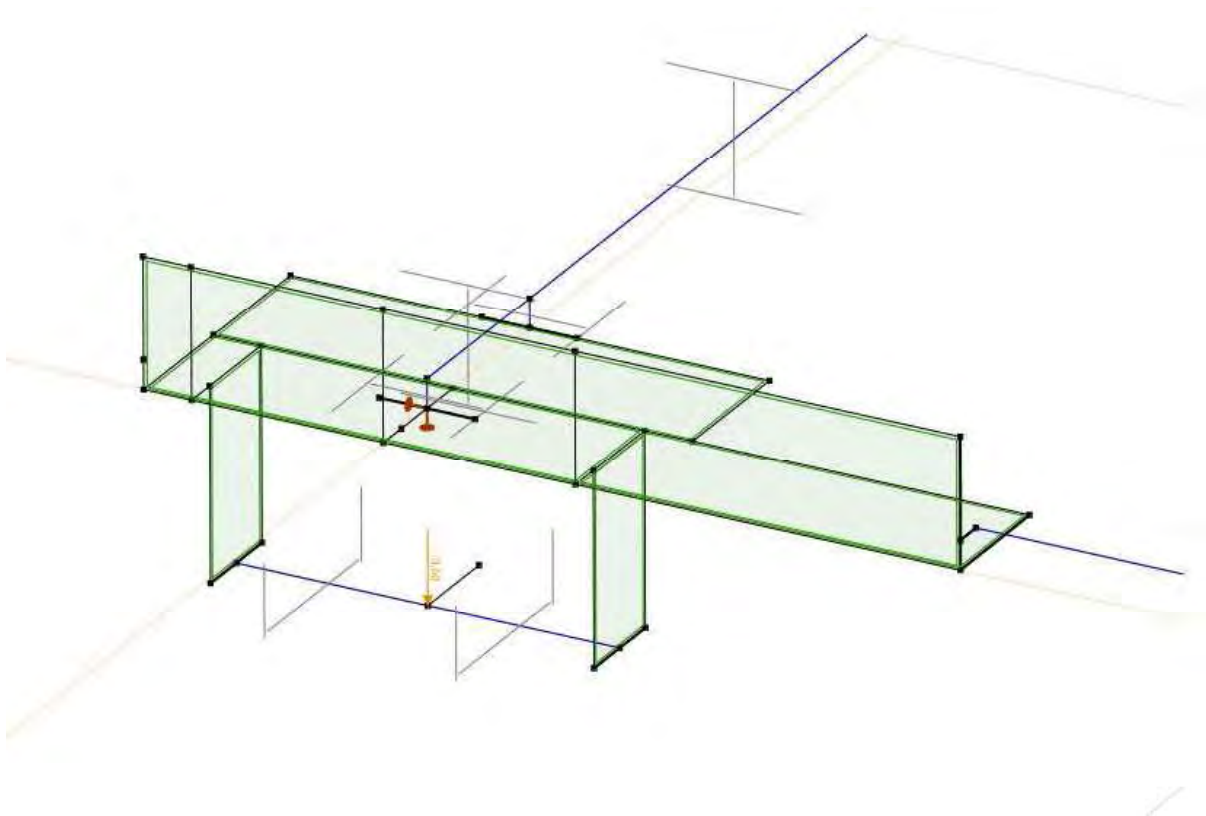
Figuur 9 Rekenmodel krachtsinleiding post-isolator aan onderrand
