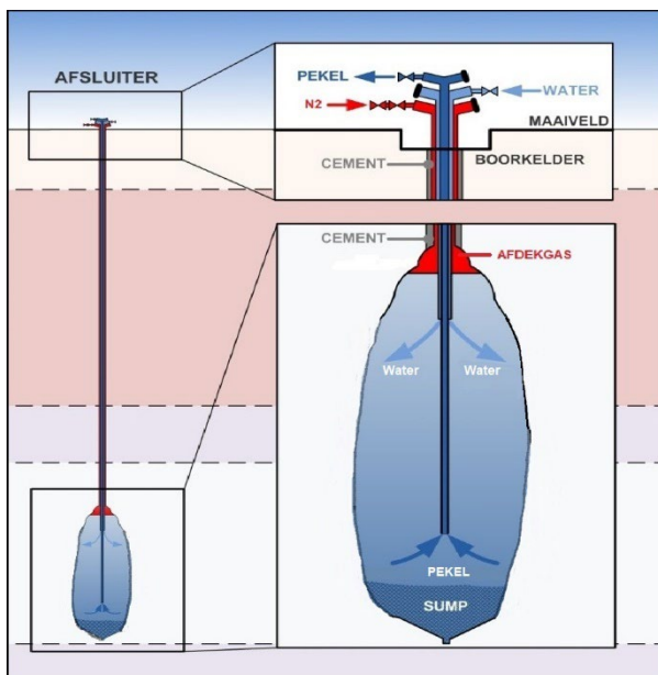
Figuur 3-5: Proces van uitloging (afgebeeld met afdekgas).
