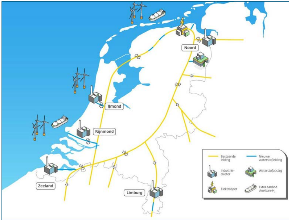
Figuur 2-2: Waterstofketen: windpark op zee, elektrolyzers, leidingen, opslag en industriële afnemers.
