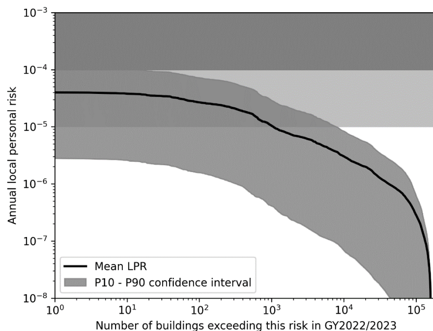
Figuur 7.1 LPR-grafiek voor gasjaar 2022/2023 voor scenario Update november 2022 met door TNO voorgestelde modelinstellingen. Op de horizontale as staat het aantal gebouwen; op de verticale as het LPR. De grafiek geeft voor elk aantal op de horizontale as de LPR-waarde van het aantal gebouwen, dat overschreden wordt. De dikke zwarte lijn geeft de verwachtingswaarde (mean) van het LPR aan. De donkergrijze band geeft de spreiding in de beslisboom voor modelonzekerheden weer voor een betrouwbaarheidsinterval van tussen percentielen P10 en P90. De twee horizontale vlakken in lichtgrijs geven het tijdelijke ( 10^{-4} ) en permanente ( 10^{-5} ) LPR-niveau van de Meijdamnorm aan.
