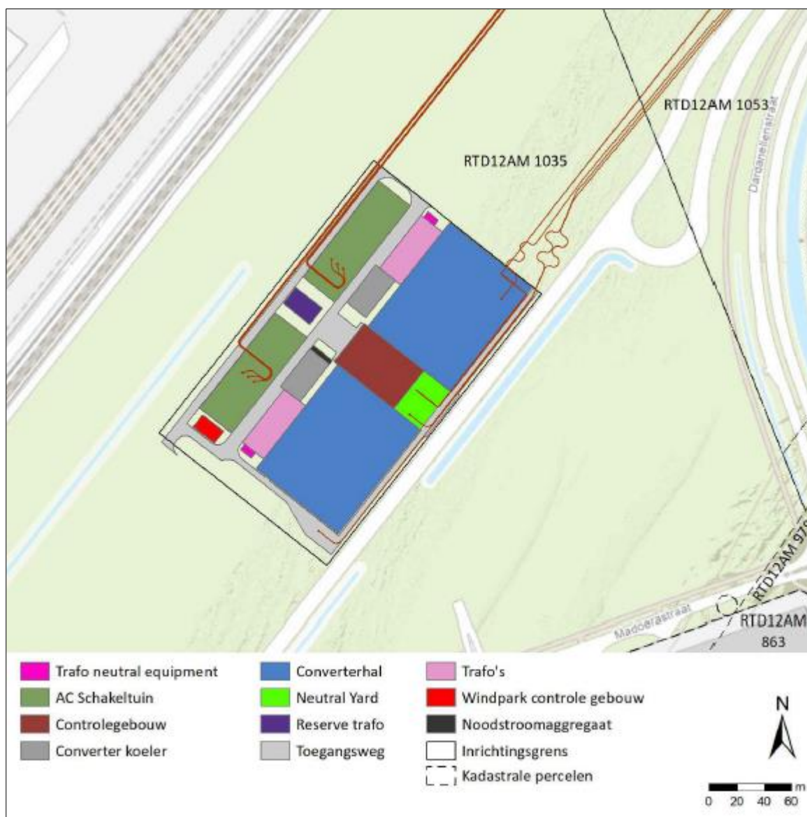
Figuur 1-2 Lay-out converterstation IJmuiden Ver Gamma op de Maasvlakte, Rotterdam
