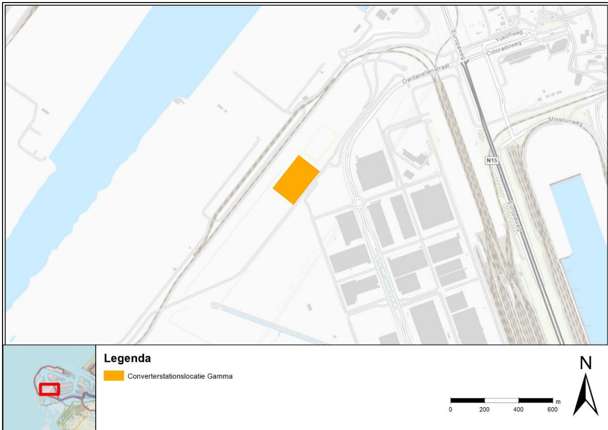
Figuur 1-1 Ligging converterstation Net op zee IJmuiden Ver Gamma
