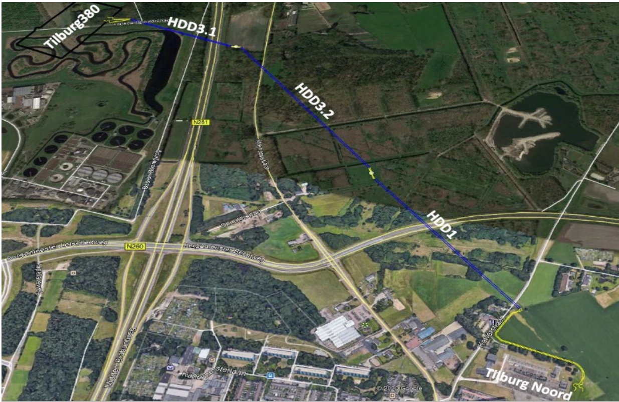
Figuur 1-3 150 kV Ondergrondse kabelroute van Tilburg 380 kV naar Tilburg Noord 150 kV
