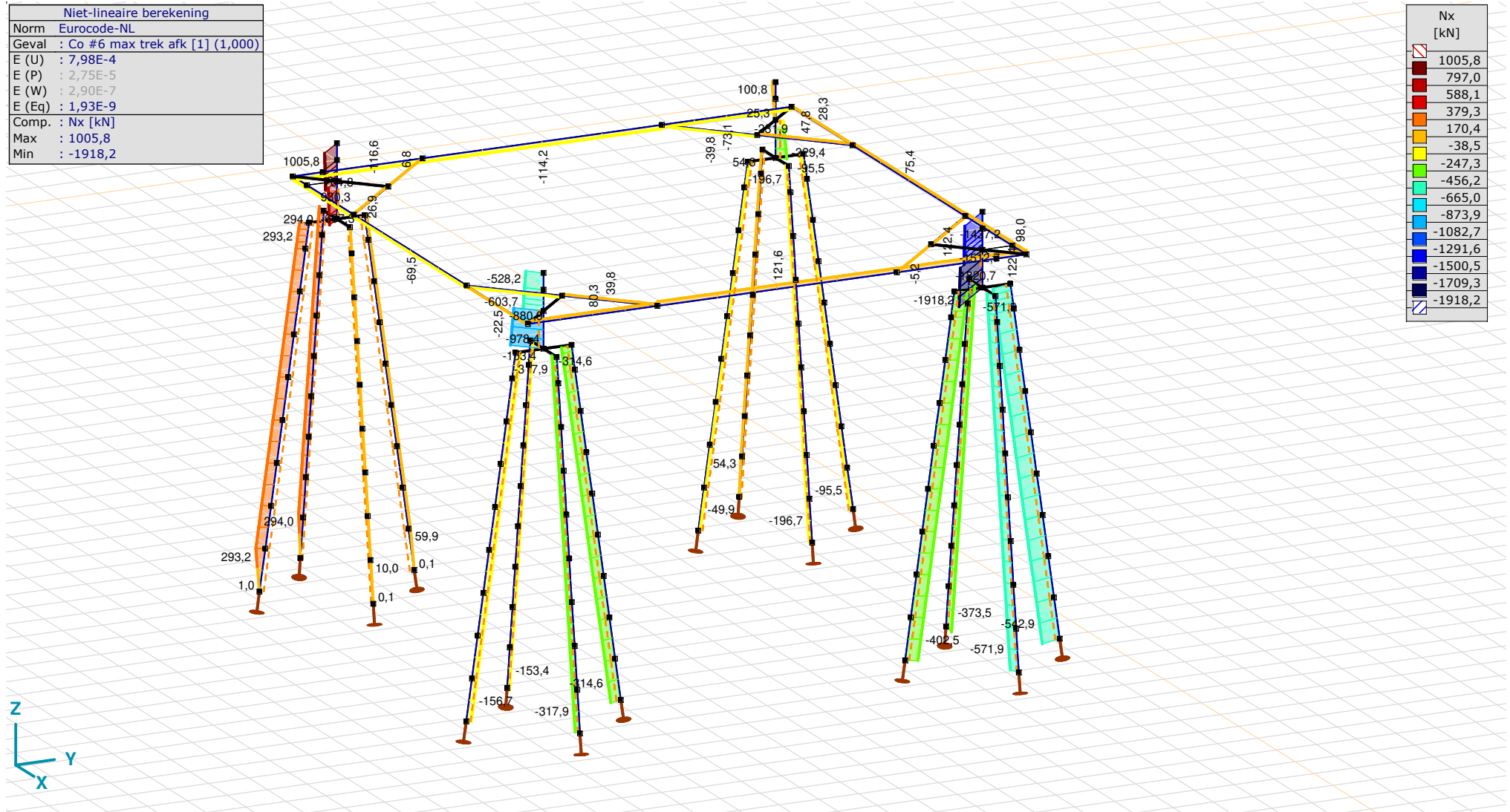
[II], Non-lin., Co #6 max trek afk [1] (1,000), Nx, Lijnen (gevuld)(gevuld)
