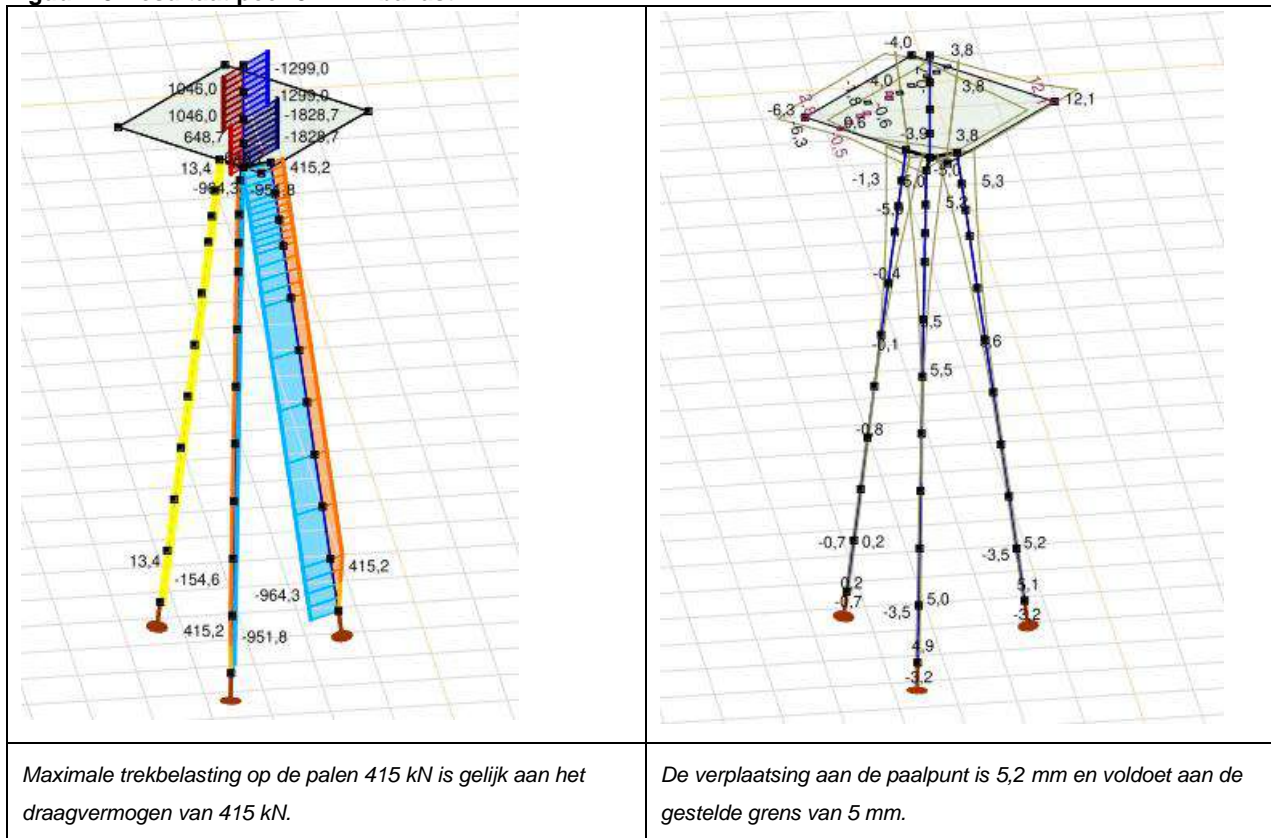
Figuur 19 Resultaat poer 3P-LD+ballast
