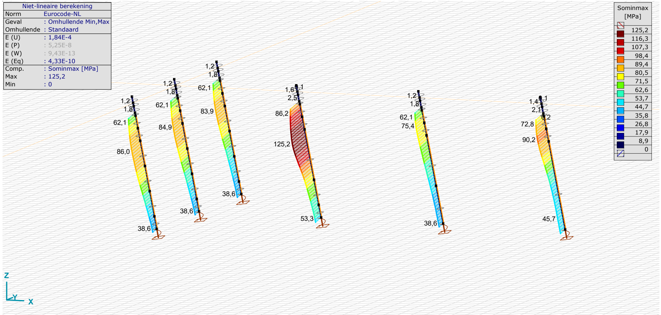
[II], Non-lin., Omhullende (Standaard), Sominmax, Lijnen (gevuld)
