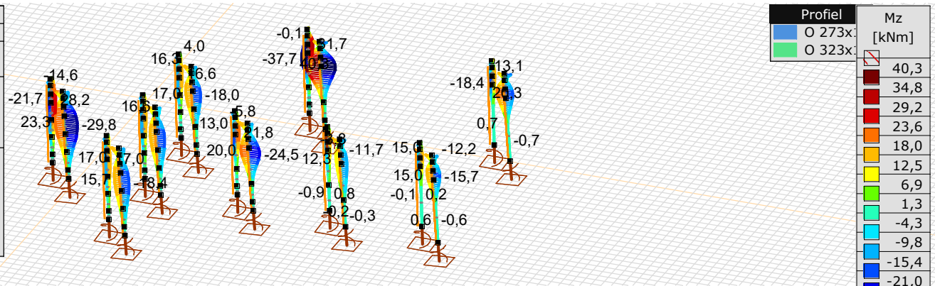
[II], > 2 details, Non-lin., Omhullende (Alle UGT ), Lijnen (gevuld), x 2
