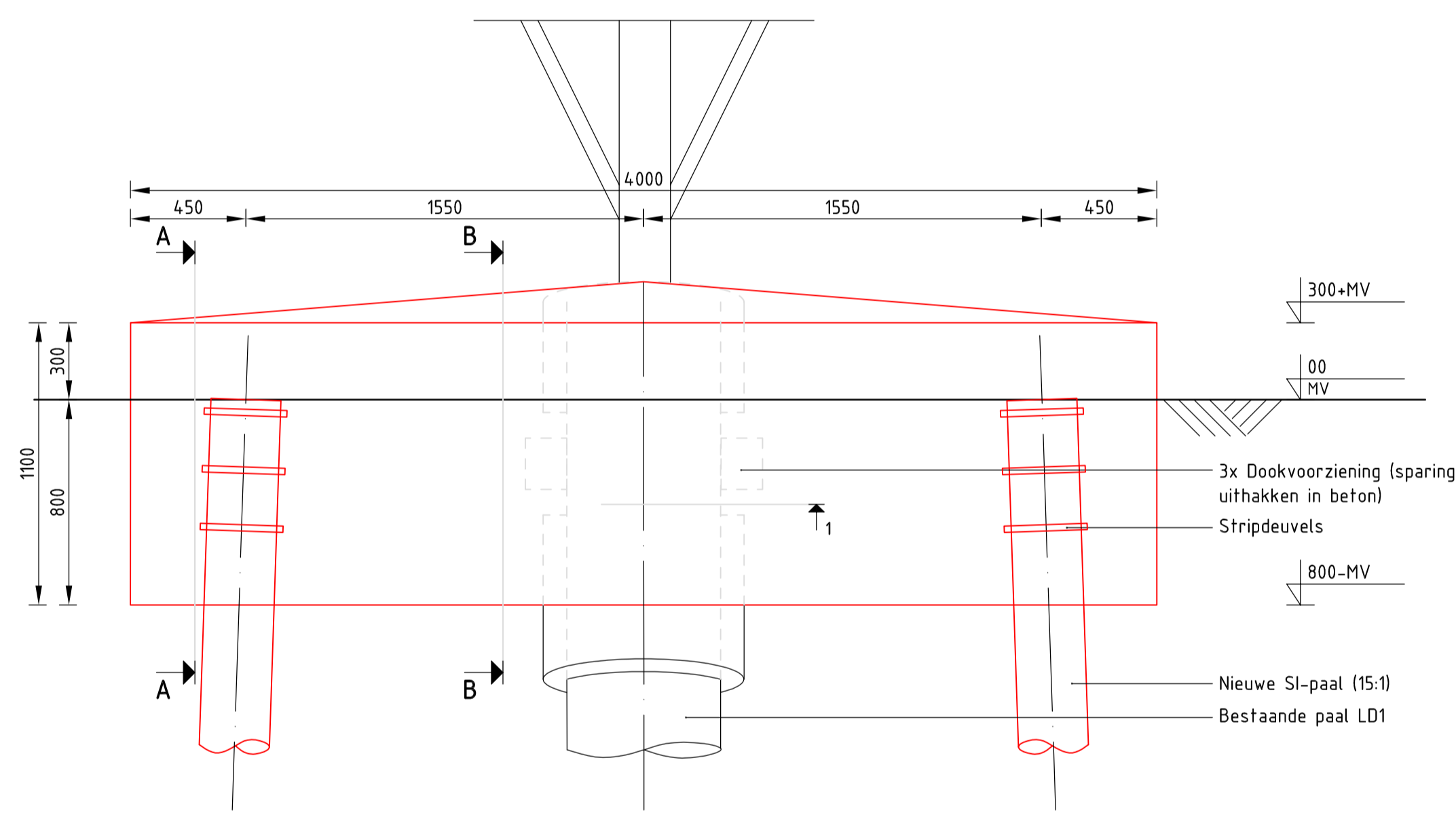
Aanzicht fundatieversterking Schaal 1:20
