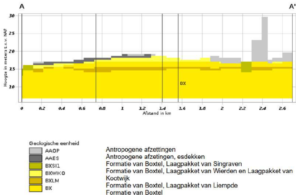
Afbeelding 2-1 Geologische doorsnede van het plangebied (Bron: Dinoloket).
