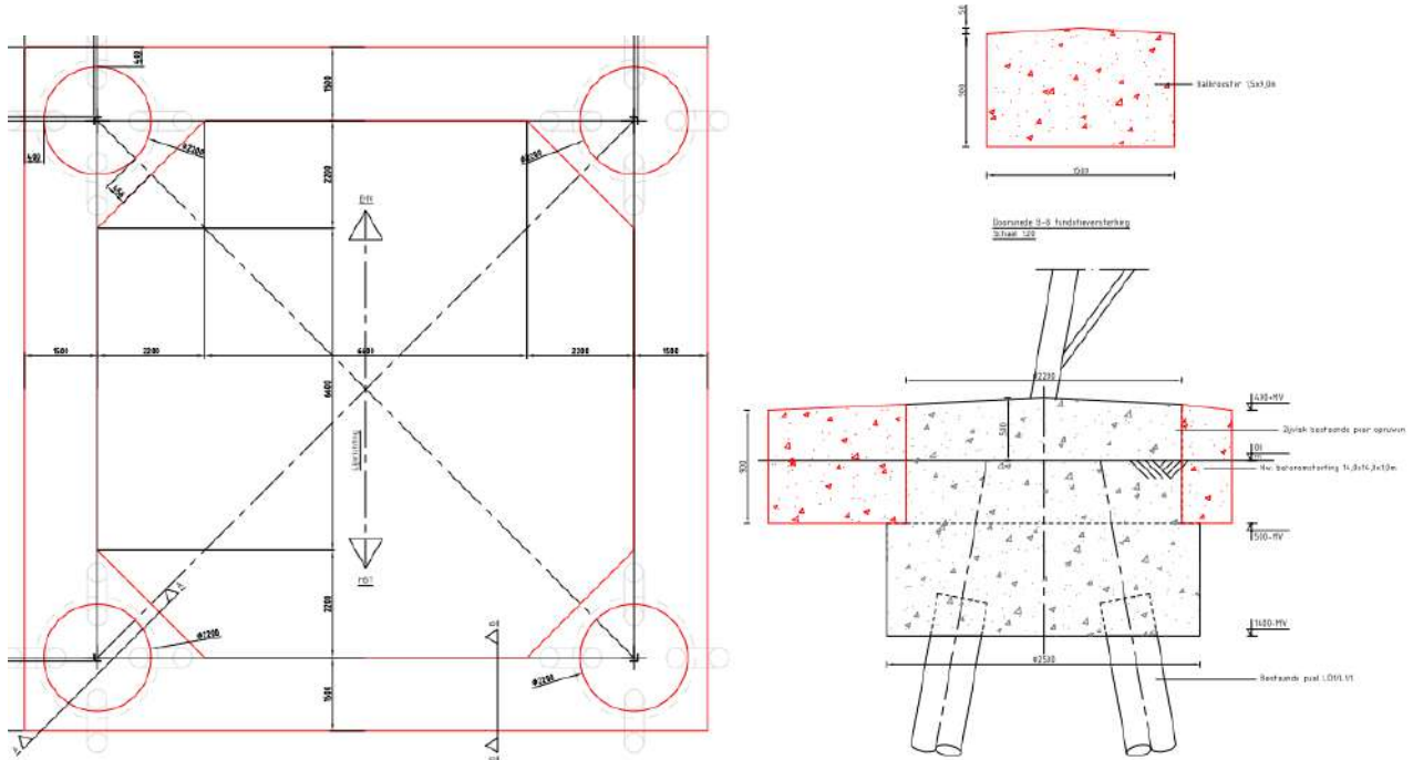
Figuur 6-2 Ballastverzwaringen - balkrooster
