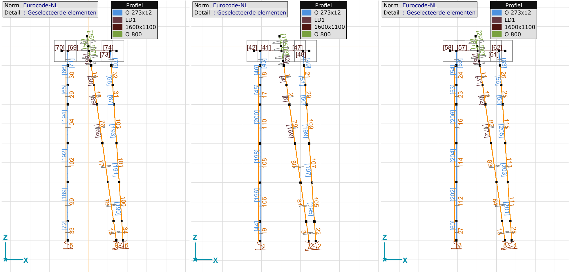
Staven en opleggingen - grondopbouw type 1 (links lage bedding, midden gemiddeld en rechts hoog)
