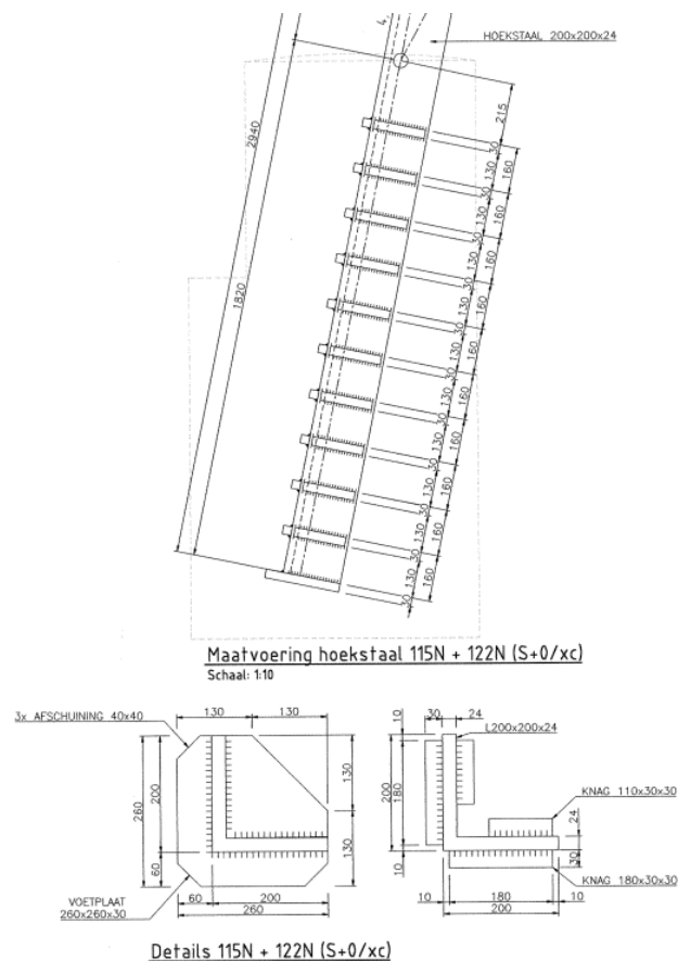
Figuur 5 Deel van de funderingstekening
