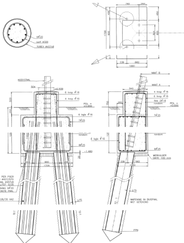
Figuur 7 Schroefinjectiepaal als fundering voor nieuwbouwmasten 115,121 en 122
