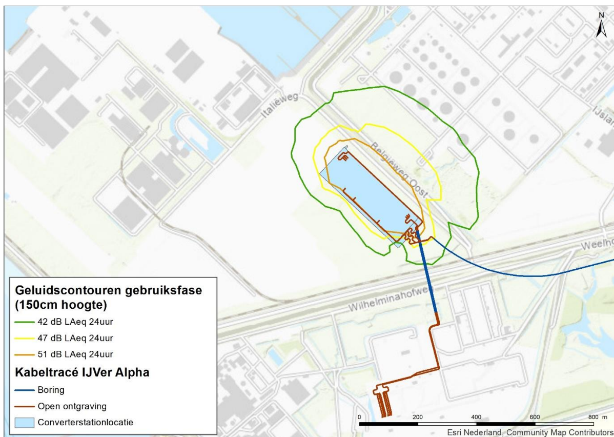
Figuur 44 Contouren van verstoringafstanden als gevolg van geluid op land rond het converterstation
