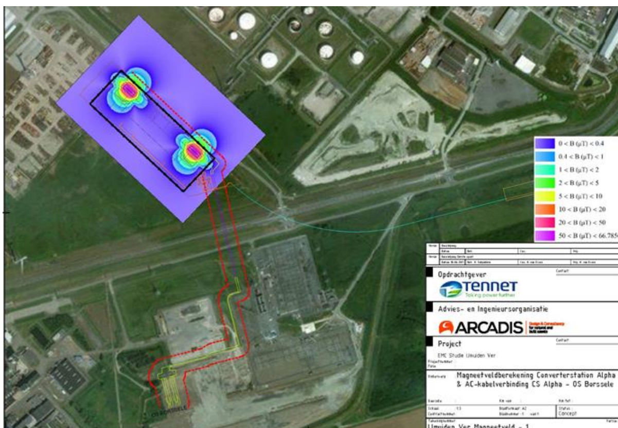
Figuur 50 Magneetveld op converterstation Alpha en bufferzone van AC-kabelverbinding converterstation Alpha-380kV-station Borssele. De rode lijnen geven de 0,4 \mu T contouren weer. Paarse en groenen lijnen de 380kV-wisselstroomverbinding die converterstation Alpha verbindt met 380kV-station Borssele, en de zwarte lijn geeft het hekwerk
