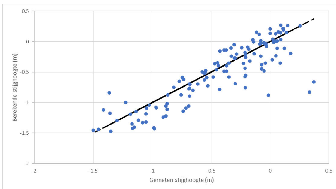
Figuur 3-8 Vergelijking gemeten versus berekende stijghoogten voor het optimalisatiemodel V8
