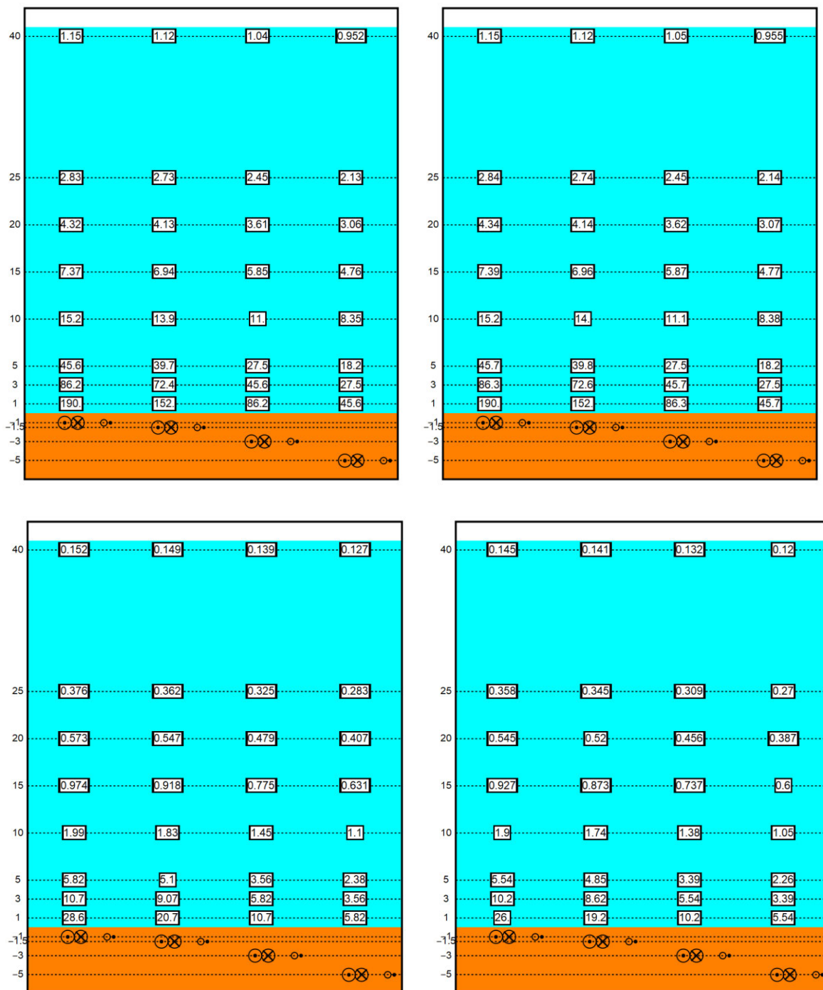
Figuur 47 Elektromagnetisch veldzone in \mu\text{T} van de 525kV-zeekabels bij een kabeldiameter van 150 (links) en 185 (rechts) mm tijdens gebruiksfase (onder) en storing/onderhoud (boven) bij de (2x2)-kabelconfiguratie. De getallen langs de verticale as zijn de begraafdiepten/meethoogten ten opzichte van het zeebodoppervlak in meter. Berekend door van Essen, 2021b.
