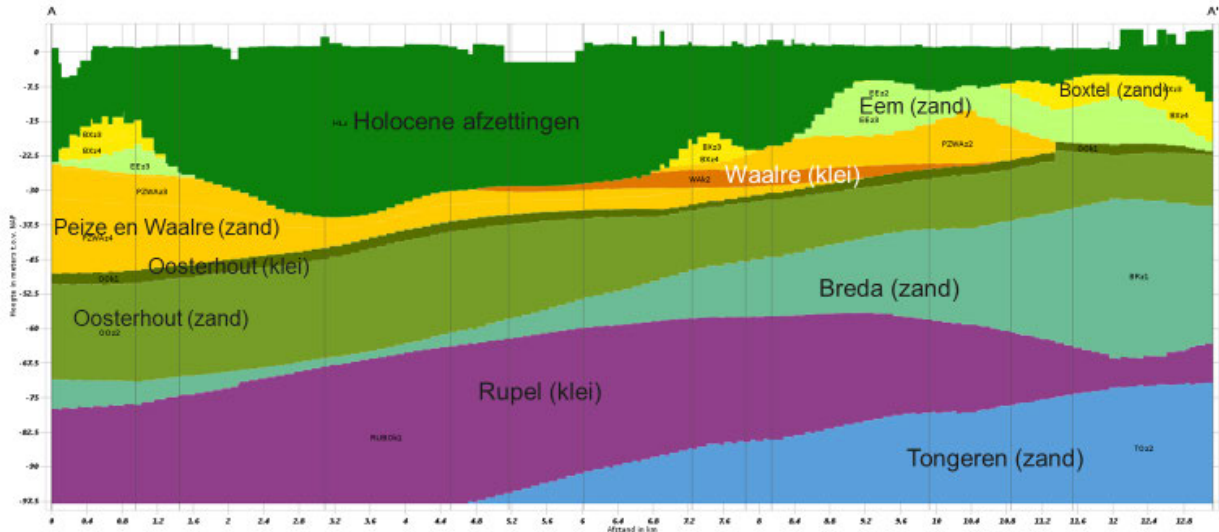
Figuur 2-3 Doorsnede van REGIS II (v2.2) van het Veerse Meer naar het converterstation te Borssele.
