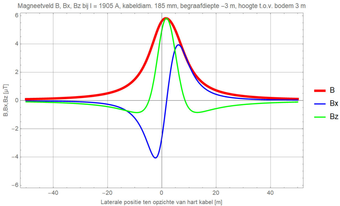
Figuur 55 (Onbalans / asymmetrie: DMR voert 10% retourstroom)
