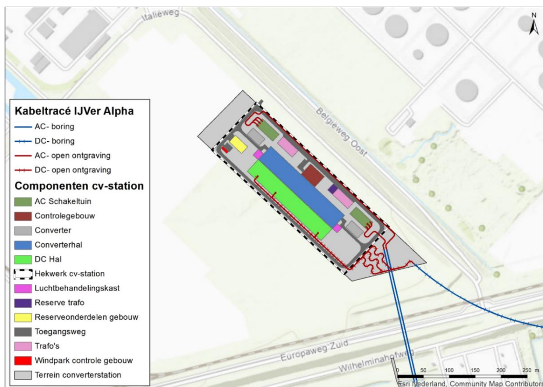
Figuur 31 Lay-out van het converterstation
