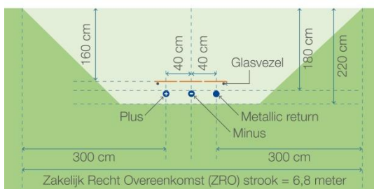
Figuur 7: Kabelconfiguratie open ontgraving IJmuiden Ver Alpha
