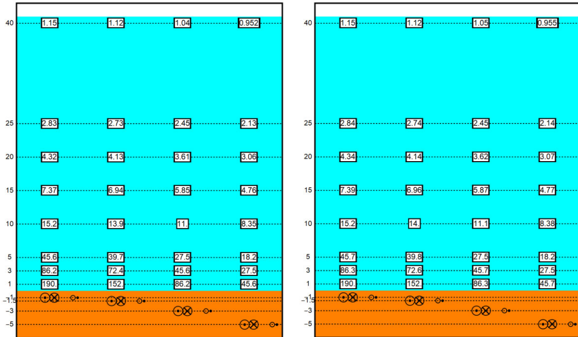
Figuur 4-14 Elektromagnetisch veldzone in \mu\text{T} van de 525kV-zeekabels bij een kabeldiameter van 150 (links) en 185 (rechts) mm tijdens storing/onderhoud bij de (2x2)-kabelconfiguratie. De getallen langs de verticale as zijn de begraafdiepten/meethoogten ten opzichte van het zeebodemoppervlak in meter. Berekend door van Essen, 2021b
