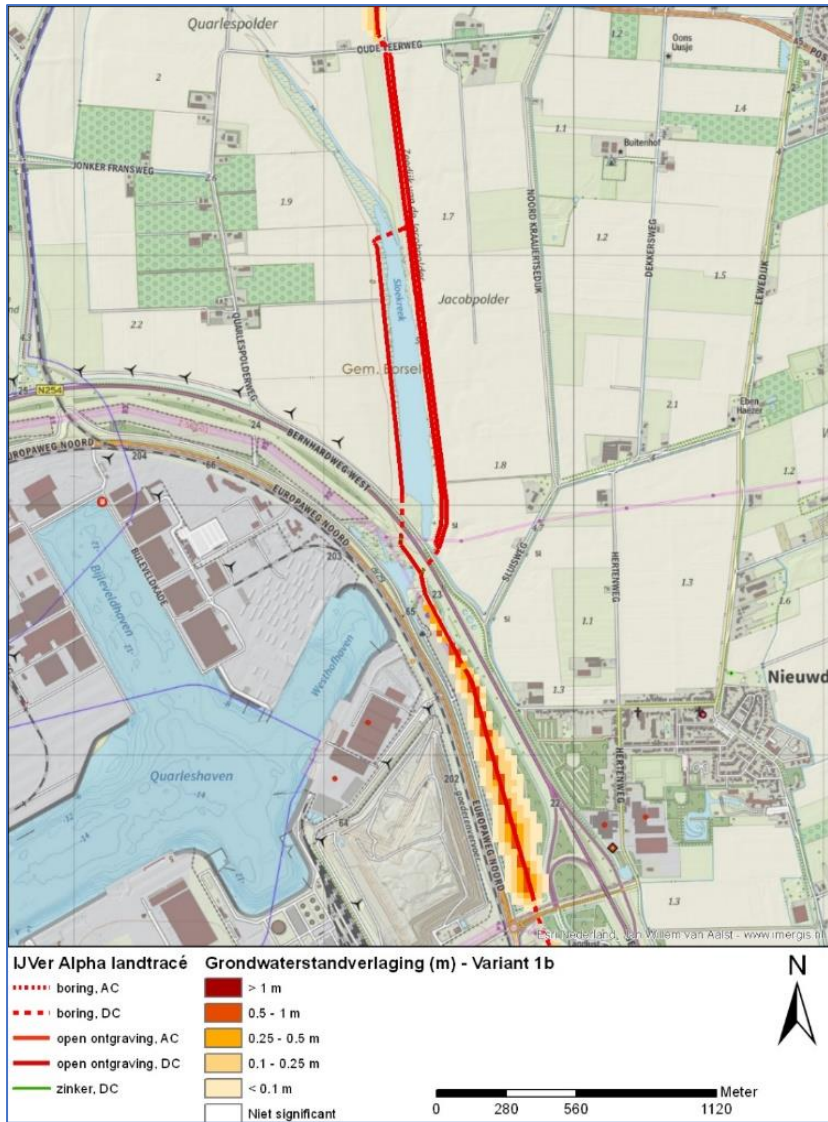
Figuur 5-4 Grondwaterstandverandering VKA-tracé - variant Sloekreek Oost dijk
