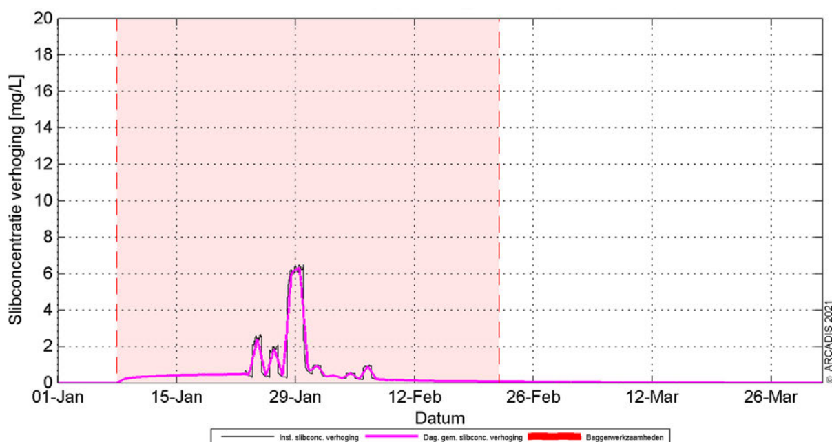
Figuur 138 Tijdsree voor de verhoging van de slibconcentratie (daggemiddelde in roze), gemeten aan het oppervlak bij stortlocatie Veere tijdens stormcondities voor scenario V1 (scenario V1 is identiek aan V2 voor stortlocatie Veere). De tijdsduur van de totale baggerwerkzaamheden in het Veerse Meer is rood gearceerd. De gebruikte startdatum van de baggerwerkzaamheden, 8 januari, is hypothetisch.
