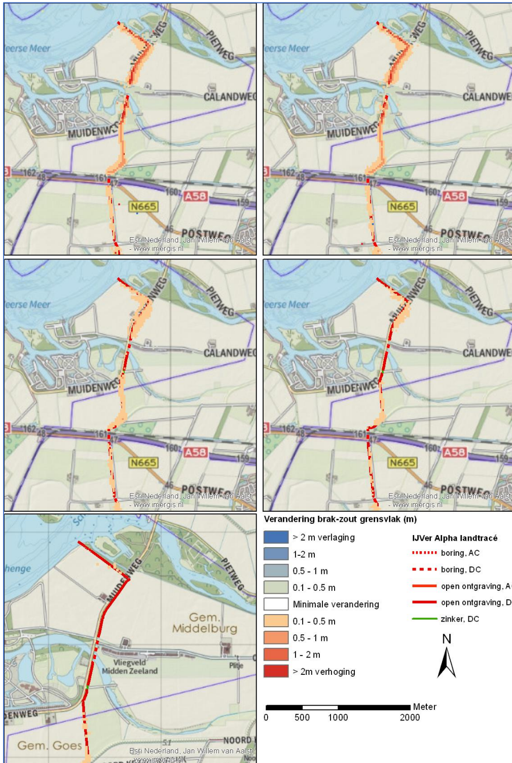
Figuur 5-27 Herstel van het brak-zout grensvlak voor het noordelijk deel van het tracé (van linksboven naar rechtsonder de jaren 0,5, 1, 5, 10 en 20 jaar)
