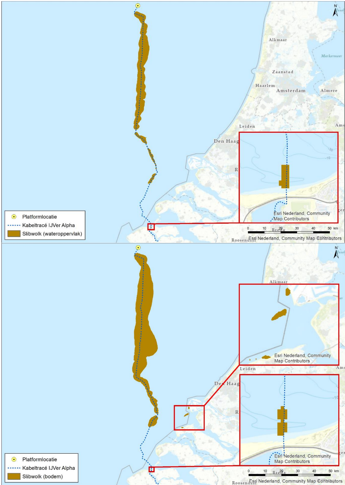
Figuur 4-1 Gebied tot waar de slibwolven aan het wateroppervlak (boven) en op de bodem (onder) (> 2 mg/l) maximaal reiken ten gevolge van de werkzaamheden
