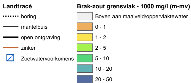
Figuur 4-8 Positie brak-zout grensvlak huidige situatie in m ten opzichte van maaiveld - centraal deel van het VKA-tracé op land
