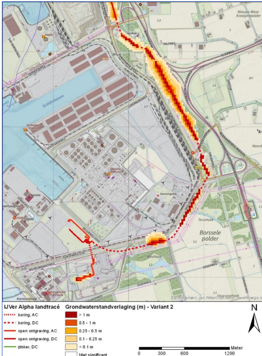
Figuur 5-6 Grondwaterstandverandering zuidelijk deel van het VKA-tracé
