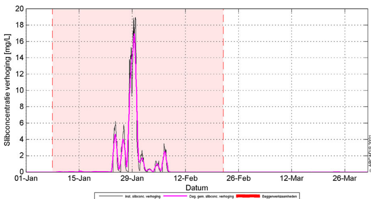
Figuur 136 Tijdsree voor de verhoging van de slibconcentratie (daggemiddelde in roze), gemeten aan het wateroppervlak bij stortlocatie Veere voor scenario V1 (scenario V1 is identiek aan V2 voor stortlocatie Veere). De tijdsduur van de totale baggerwerkzaamheden in het Veerse Meer is rood gearceerd. De gebruikte startdatum van de baggerwerkzaamheden, 8 januari, is hypothetisch.
