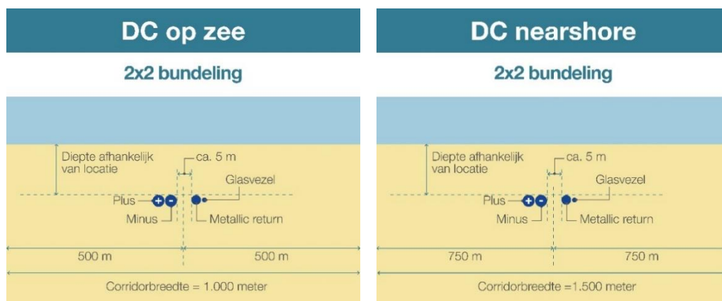
Figuur 16 Corridorbreedte (2x2)-kabelconfiguratie op zee (links) en nabij de kust (rechts)
