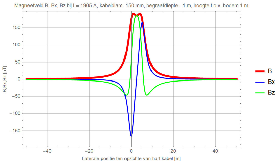
Figuur 70 (Storing / onderhoud, monopoolbedrijf: DMR voert 100% retourstroom)
