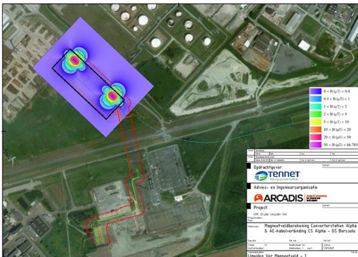
Figuur 4-17 Magneetveld op converterstation Alpha en bufferzone van AC-kabelverbinding converterstation Alpha-380kV-station Borssele. De rode lijnen geven de 0,4 \mu T contouren weer. Paarse en groenen lijnen geven de 380kV-wisselstroomverbinding die converterstation Alpha verbindt met 380kV-station Borssele. De zwarte lijn geeft het hekwerk weer.
