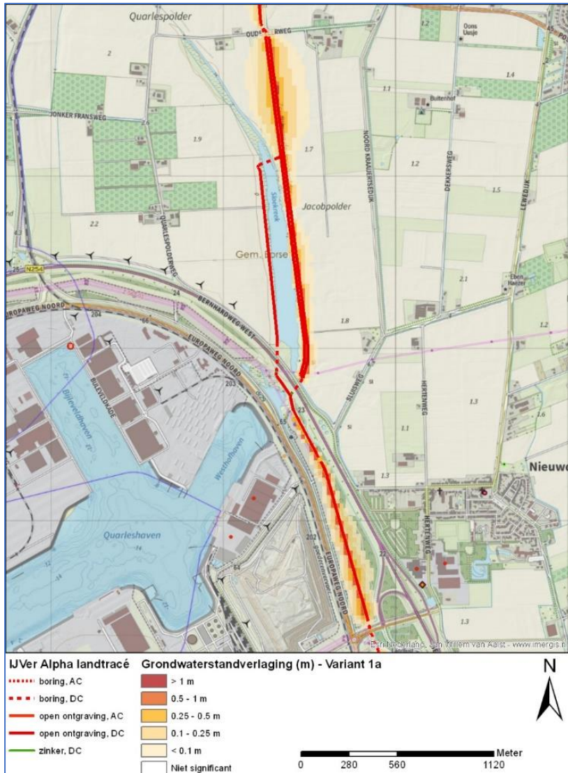
Figuur 5-3 Grondwaterstandverandering VKA-tracé - variant Sloekreek Oost Polder
