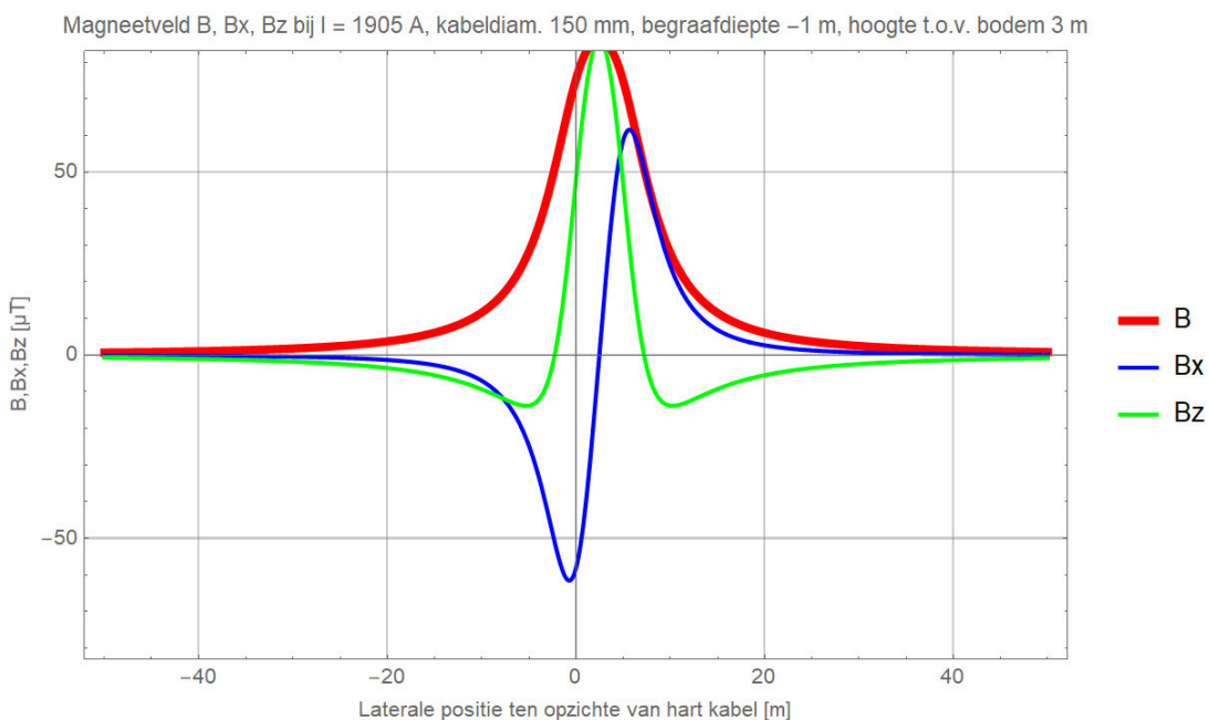
Figuur 71 (Storing / onderhoud, monopoolbedrijf: DMR voert 100% retourstroom)
