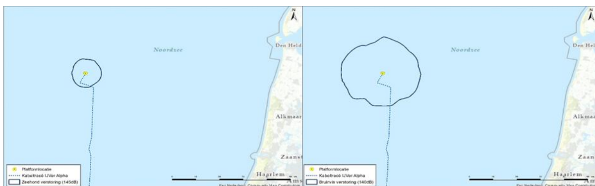
Figuur 40 Reikwijdte van onderwaterverstoring als gevolg van impuls-onderwatergeluid voor het heien van de fundering van het platform Net op zee IJmuiden (in het geval van een stalen jacket), voor zeehonden (links) en bruinvissen (rechts)
