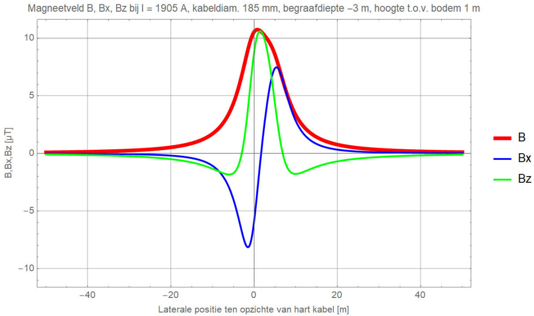
Figuur 54 (Onbalans / asymmetrie: DMR voert 10% retourstroom)
