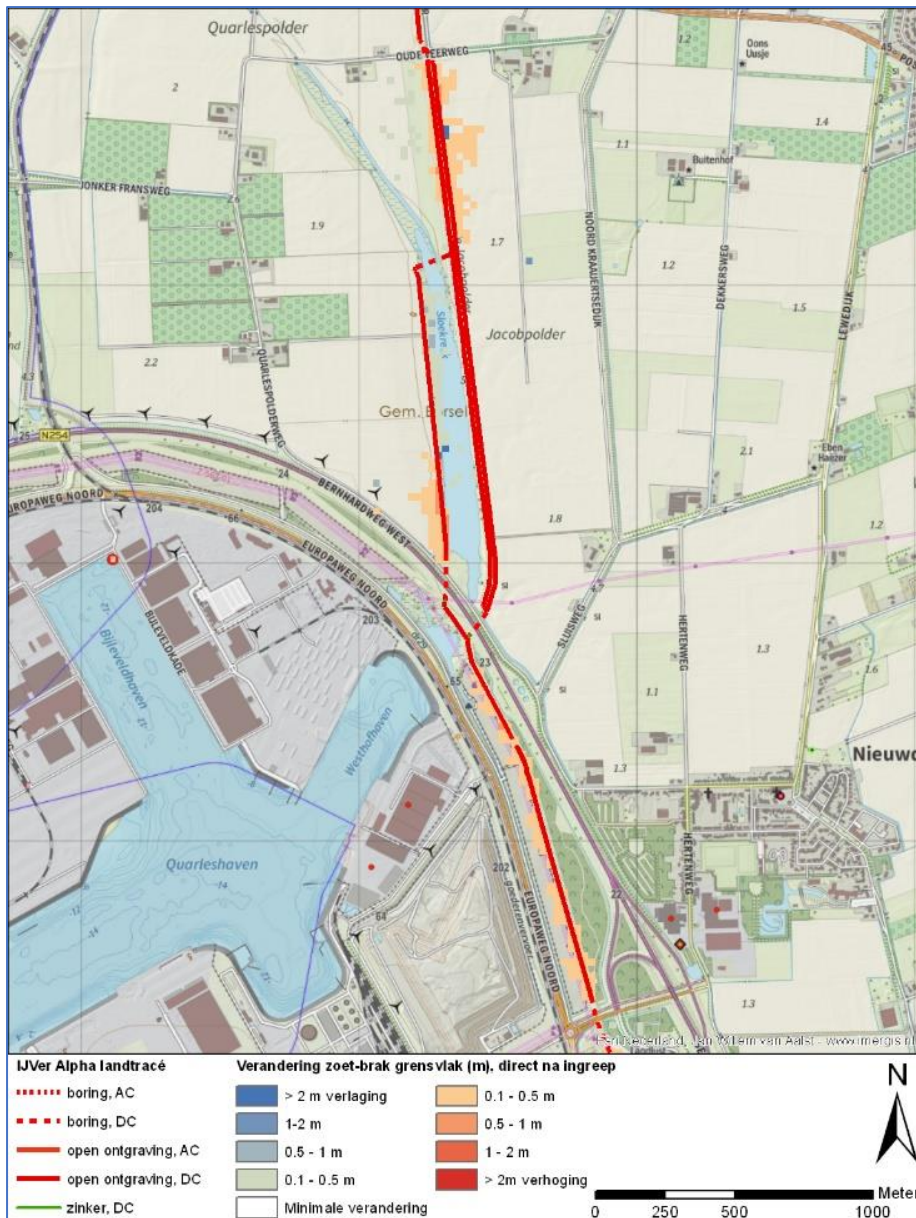
Figuur 5-10 Verschuiving zout-brak grensvlak VKA-tracé – variant west, centraal deel van het VKA-tracé op land
