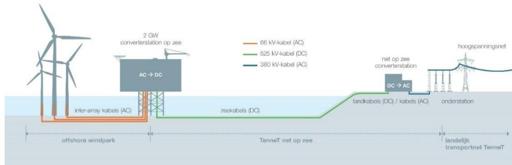
Figuur 1 Globale weergave Net op zee IJmuiden Ver Alpha
