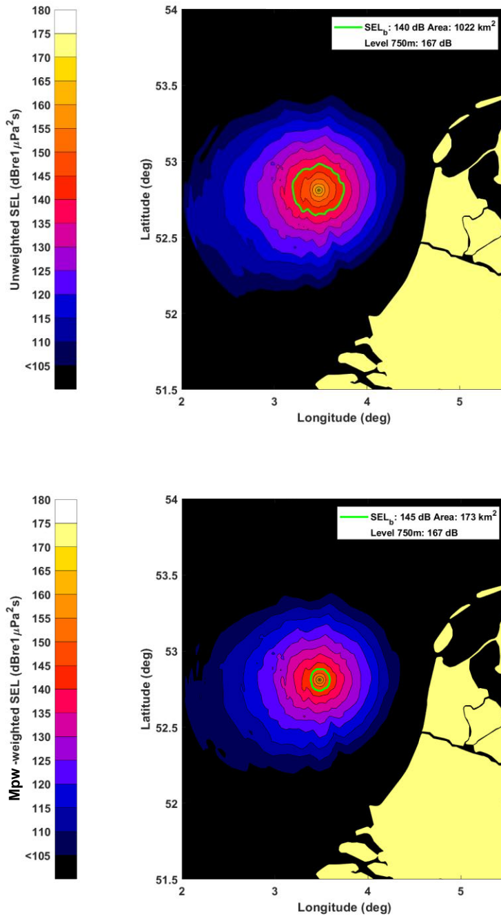
Figuur 2 Met Aquarius 4 berekende geluidskaarten (SELs) en verstoringscontouren voor bruinvissen (boven) en zeehonden (onder) voor het heien van de fundering voor het Alpha-platform voor de IJmuiden Ver windparken.
