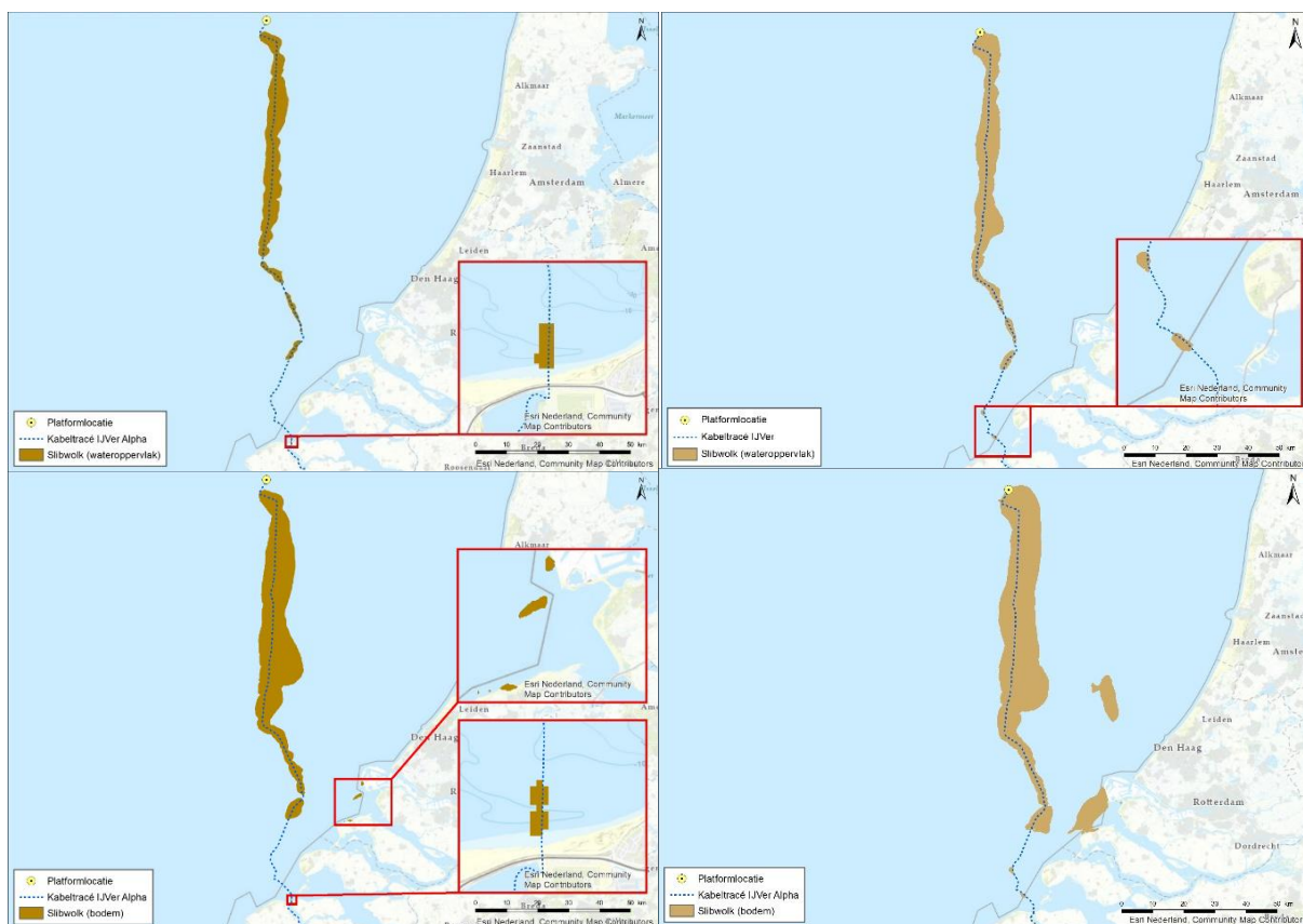
Figuur 33 Het gebied tot waar de sliwolven aan het wateroppervlak (boven) en op de bodem (onder) (> 2 mg/L) maximaal reiken ten gevolge van de werkzaamheden voor de (1x4)-kabelconfiguratie (links) en de (2x2)-kabelconfiguratie (rechts).
