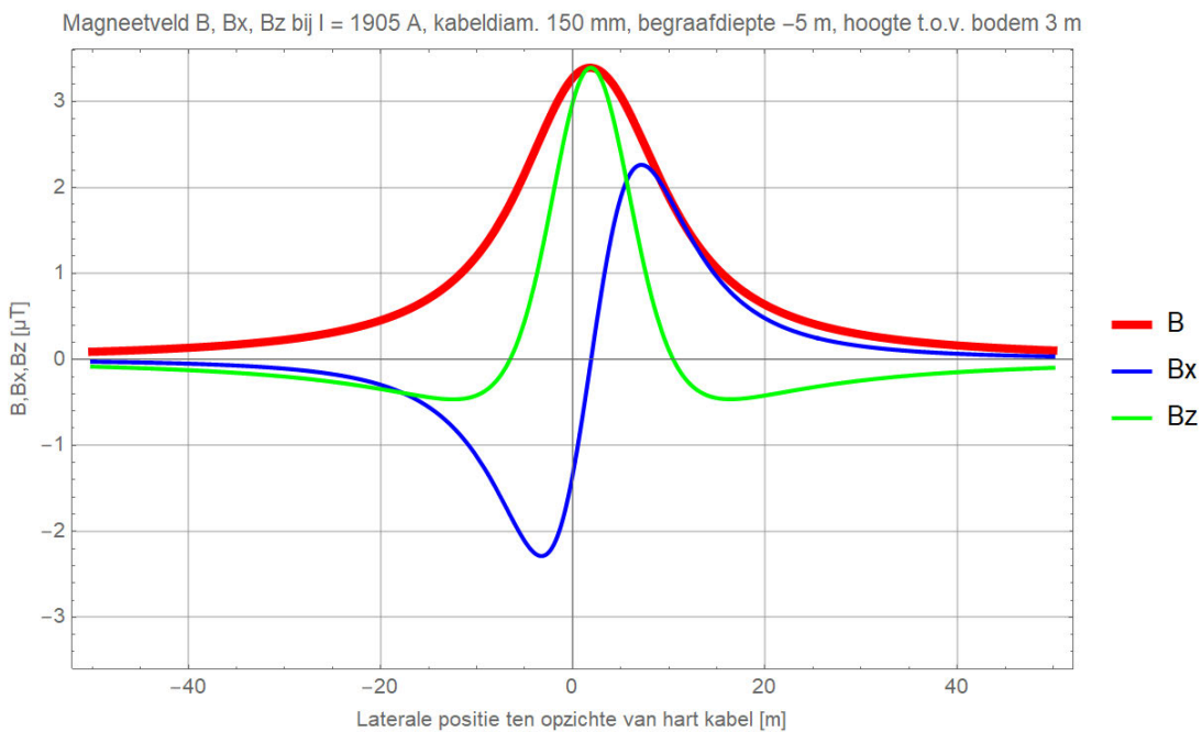
Figuur 31 (Onbalans / asymmetrie: DMR voert 10% retourstroom)
