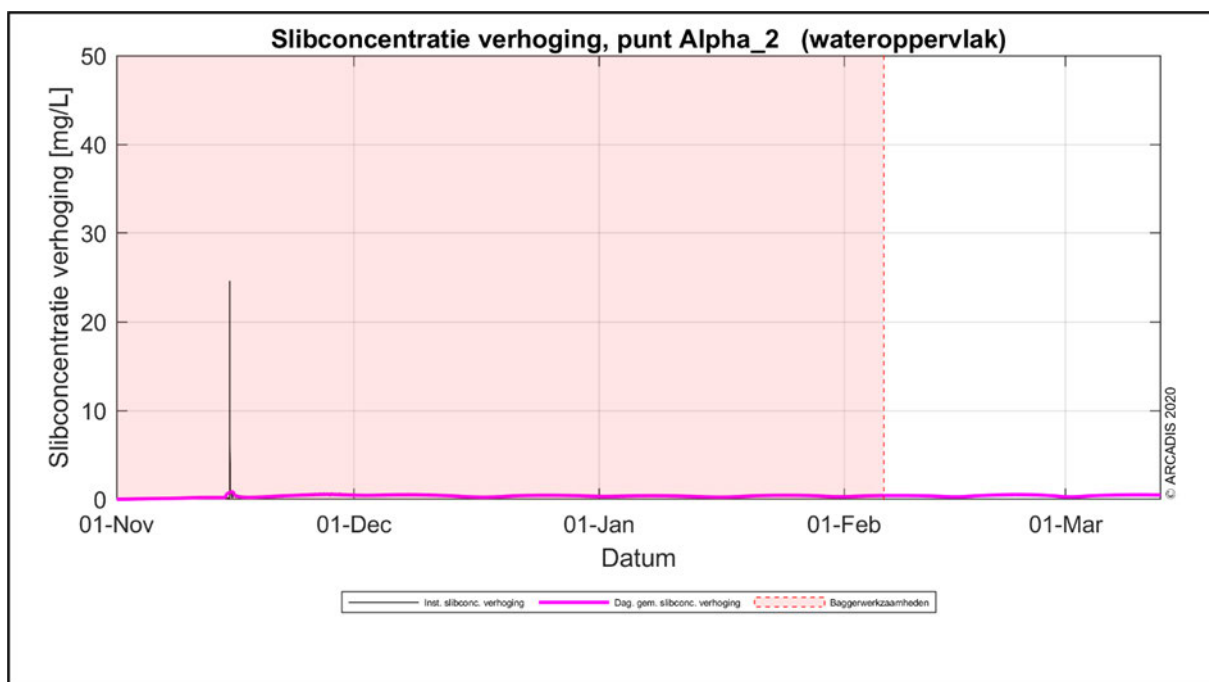
Figuur 127 Slibconcentratie aan het wateroppervlak in de tijd op punt 2
