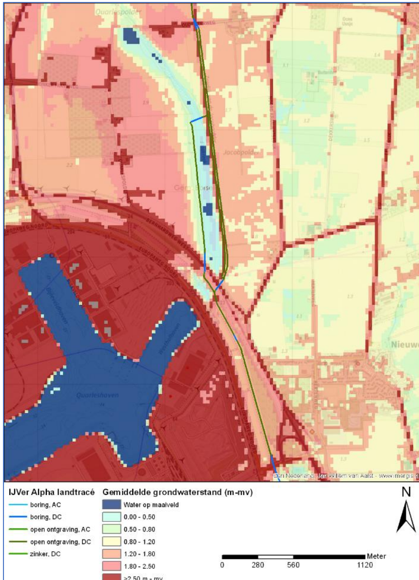
Figuur 4-2 Grondwaterstanden huidige situatie ten opzichte van maaienveld - centraal deel van het VKA-tracé op land
