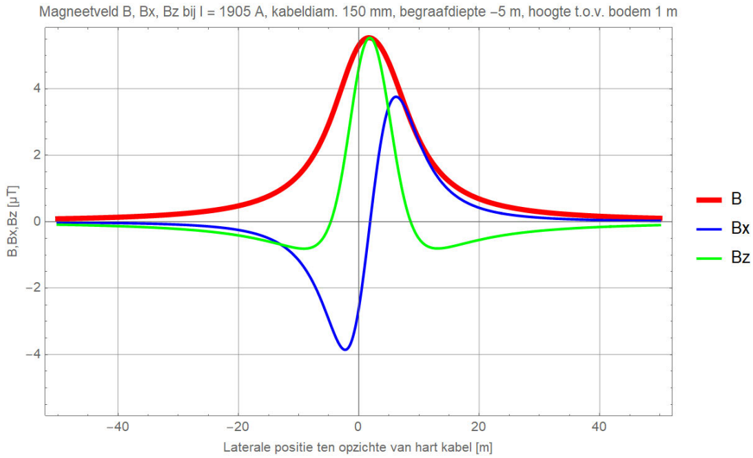
Figuur 30 (Onbalans / asymmetrie: DMR voert 10% retourstroom)
