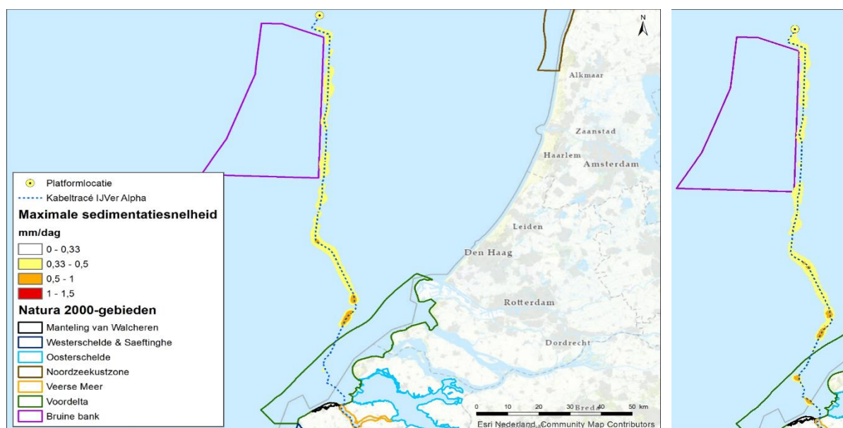
Figuur 139 Maximale sedimentatie snelheden (in mm/dag) die optreden door de werkzaamheden ten opzichte van de Natura 2000-gebieden voor de (1x4)-kabelconfiguratie (links) en (2x2)-kabelconfiguratie (rechts)
