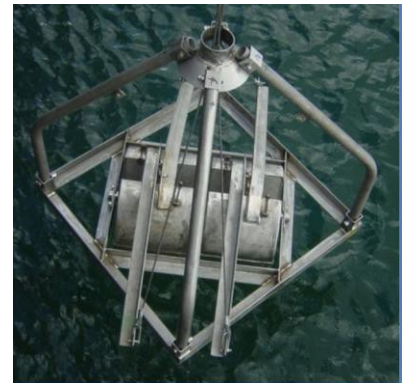
BSL-Doppelgreifer
