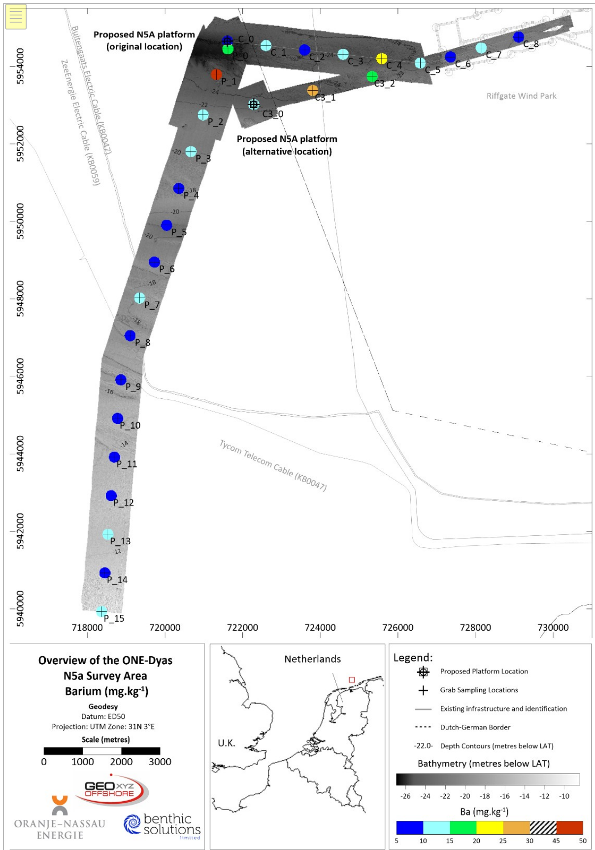
Abbildung 24: Schwermetallkonzentration für Barium (Ba; mg.kg -1 )
