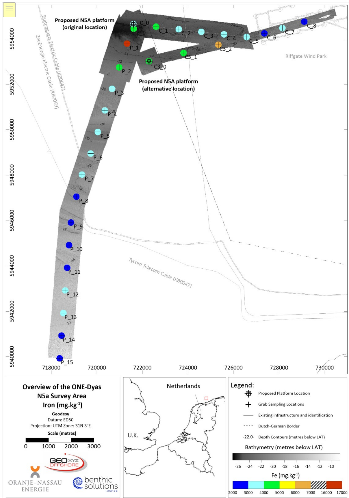
Abbildung 27: Schwermetallkonzentration für Eisen (Fe; mg.kg -1 )
