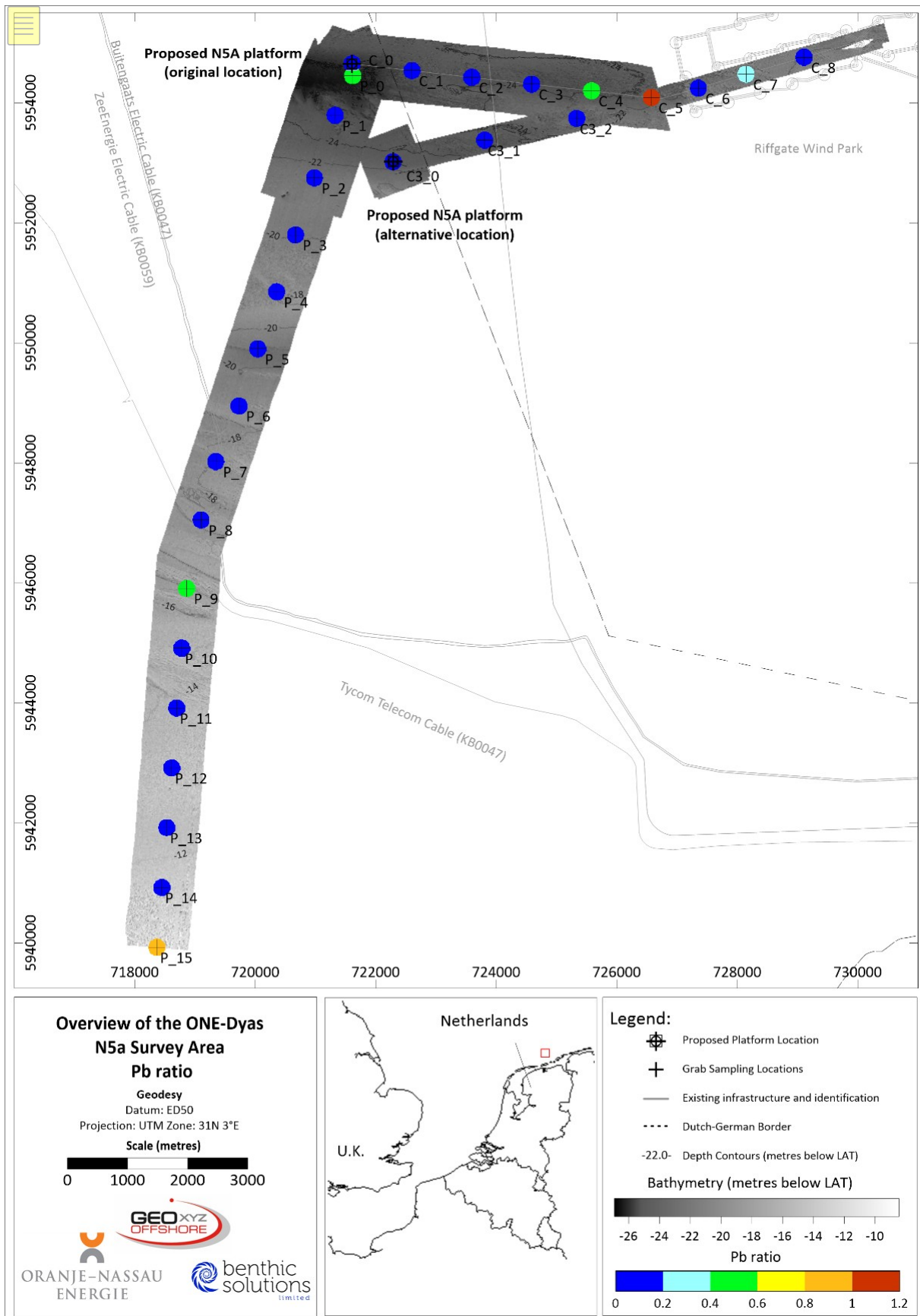
Abbildung 21: Petrogenes/biogenes Verhältnis
