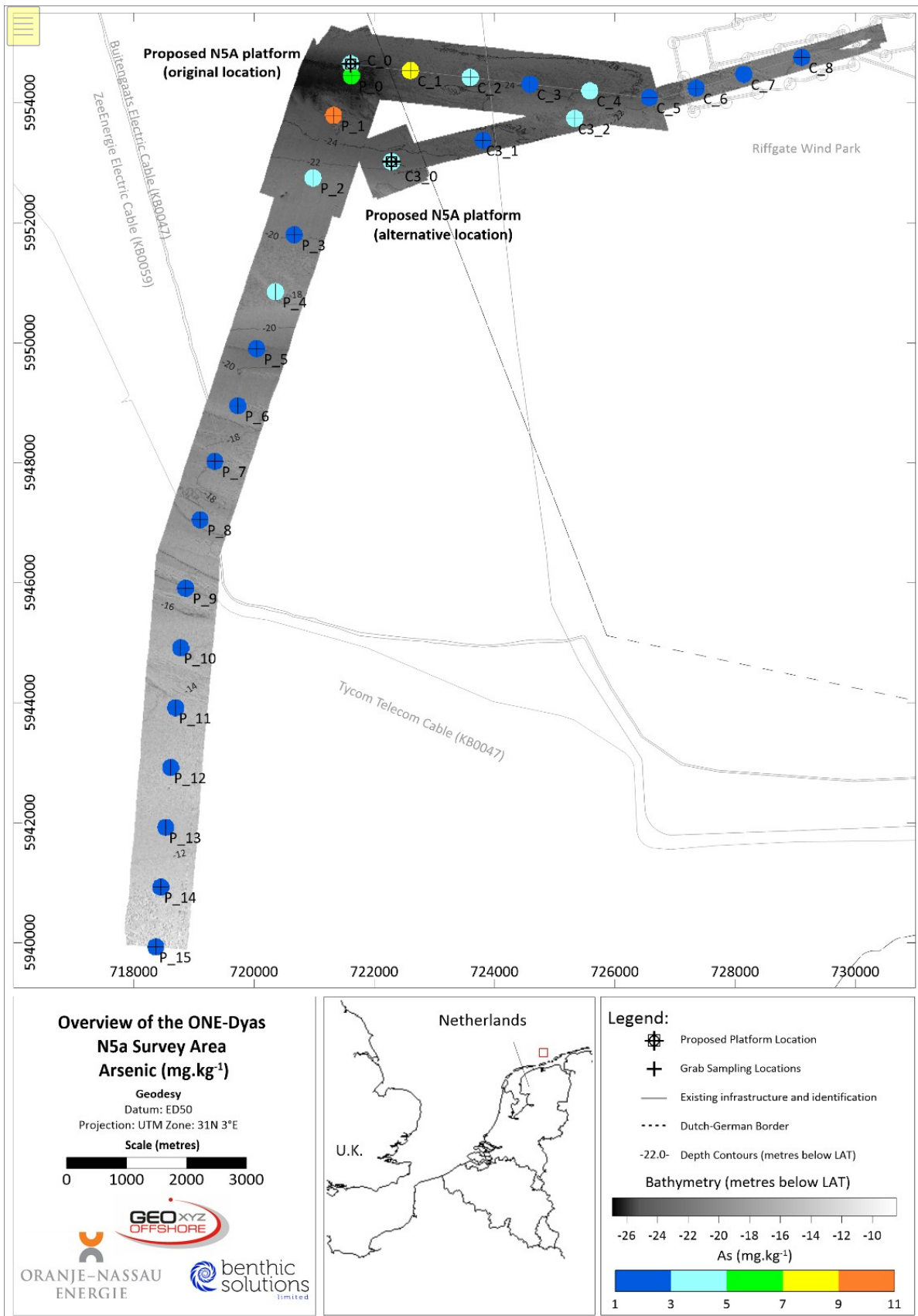
Abbildung 28: Schwermetallkonzentration für Arsen ( \text{As} ; \text{mg.kg}^{-1} )
