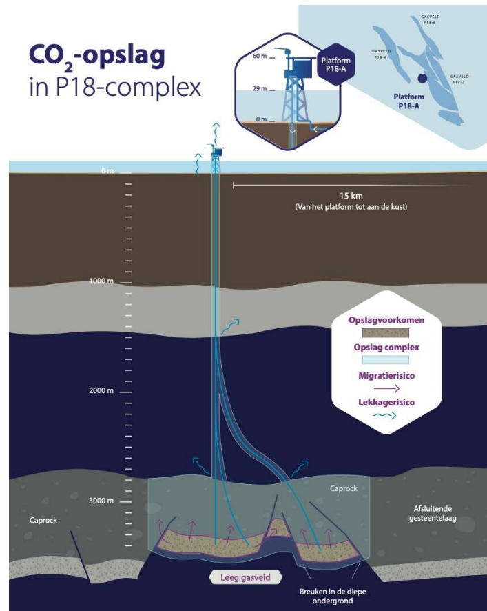
Figuur 3 Schematische weergave van de definities van opslagvoorkomen en CO 2 -opslagcomplex en de daarmee samenhangende risico's van migratie en lekkage. Belangrijk: in dit figuur wordt het P18-2 Opslagvoorkomen en -complex weergegeven, en als zodanig is deze figuur dus illustratief voor P18-4.
