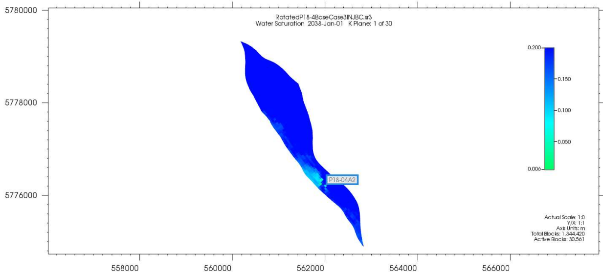
Figuur 20 Waterverzadigingsprofiel met verdampt water bij het CO 2 -koudefront.
