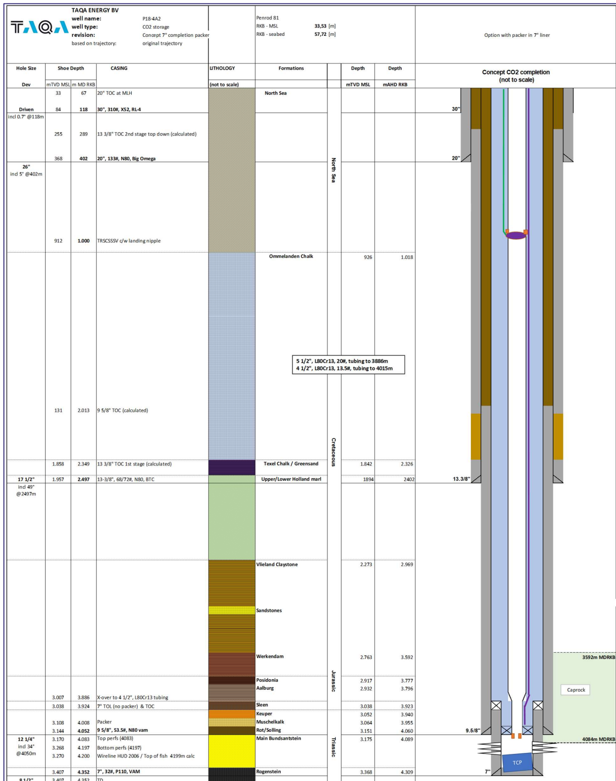
Figuur 27 Gereviseerd putontwerp voor put P18-4A2.
