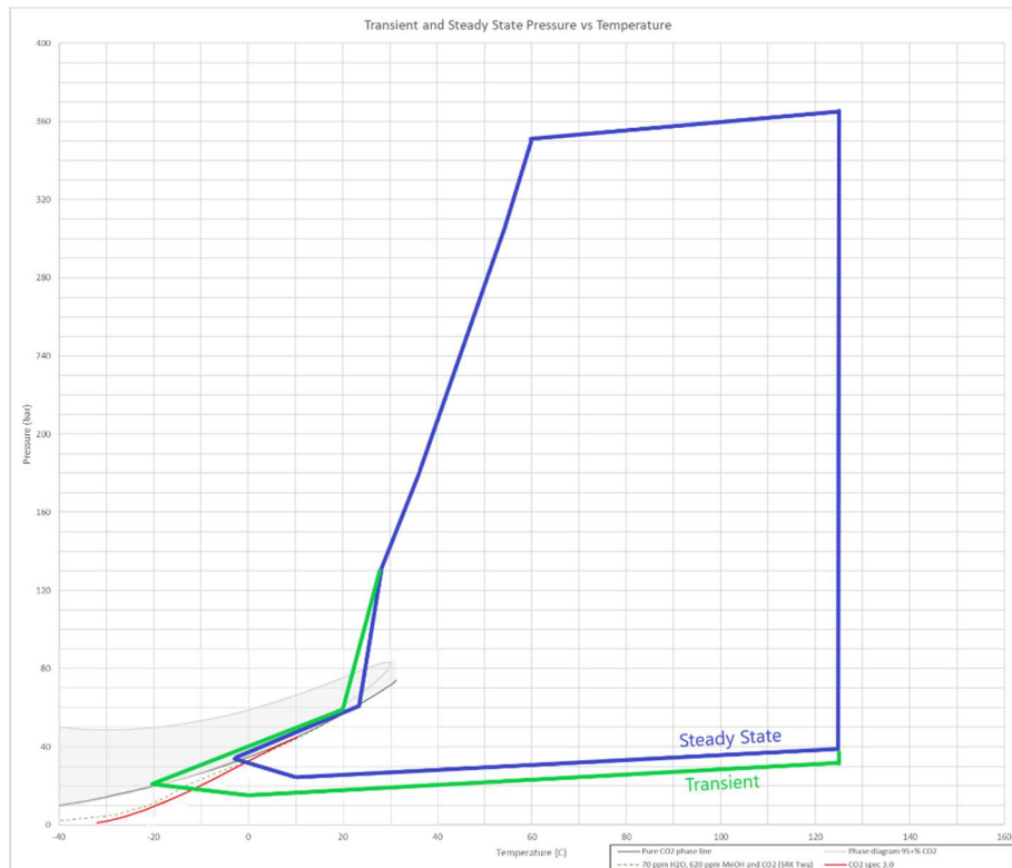
Figuur 26 Operationeel bereik van de P18 CO 2 injectieputten.
