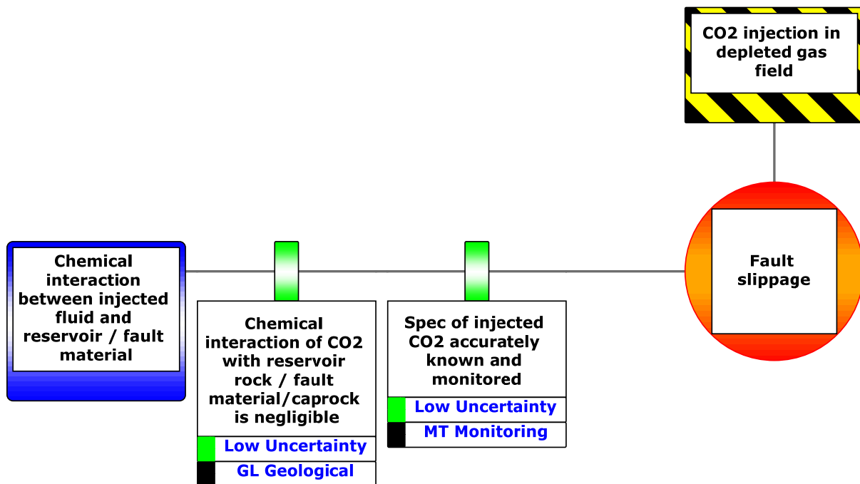
Figuur 56 Overzicht van preventieve barrières tegen chemische interactie tussen vloeistof en gesteente met breukbeweging tot gevolg.
