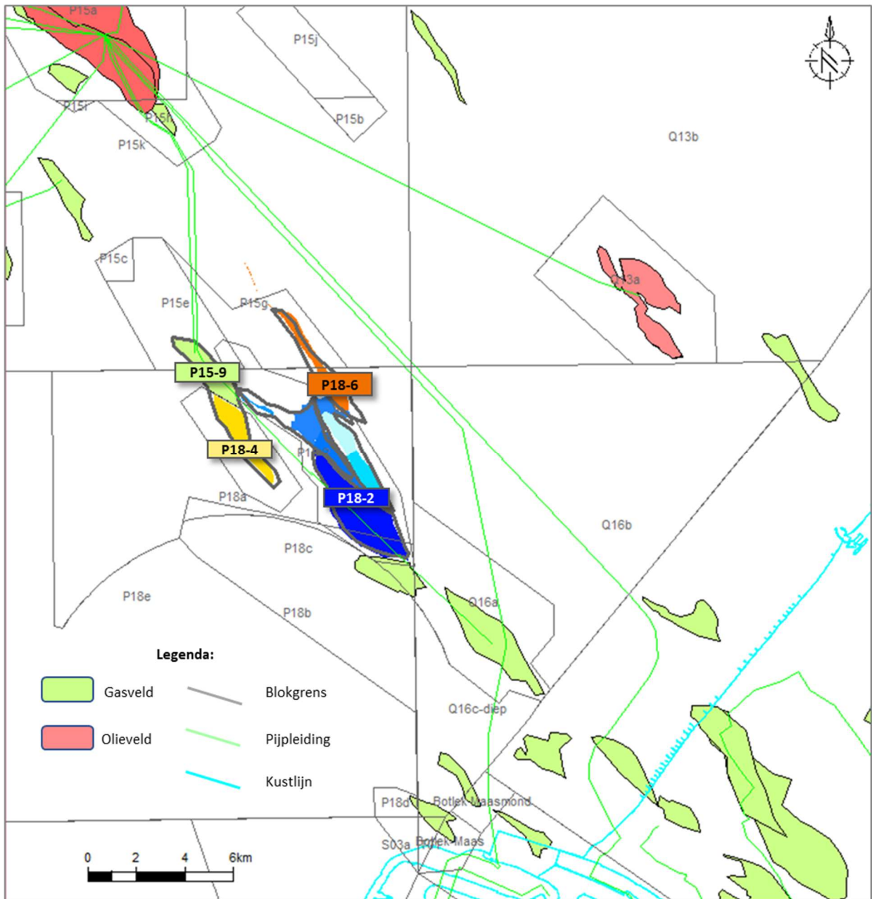
Figuur 1 Kaart van Blok P18 en directe omgeving. De P18-reservoirs bevinden zich grotendeels in Blok P18 en deels in Blok P15 en beslaan de huidige P18a, P18c en P15g winningsvergunningen, en ook de Opslagvergunning P18-4. De reservoirs P15 en P18 zijn aangegeven in kleuren overeenkomstig met de overige reservoirkaarten in dit document. Zie legenda voor de verklaring van de overige symbolen.
