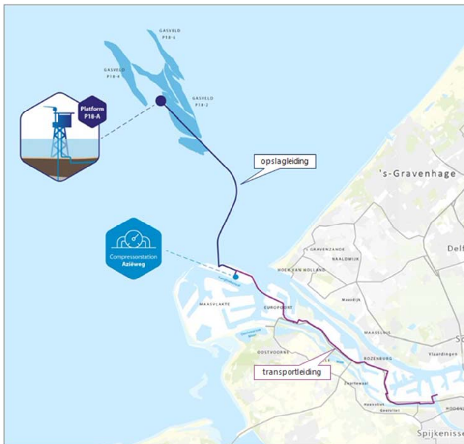
Figuur 3 Overzicht van het Porthos Systeem.
