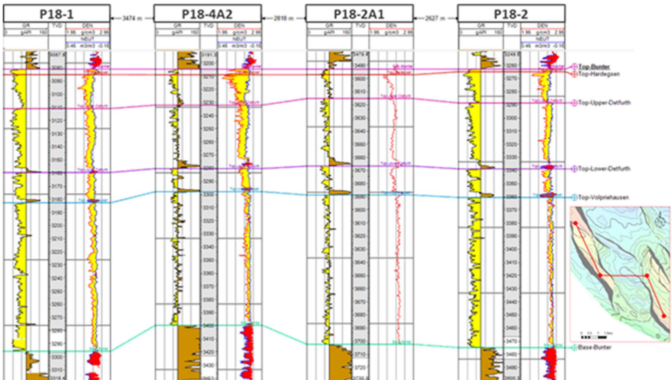
Figuur 12 Boorlogcorrelatie door reservoir P18-4 met verbinding naar P18-2
