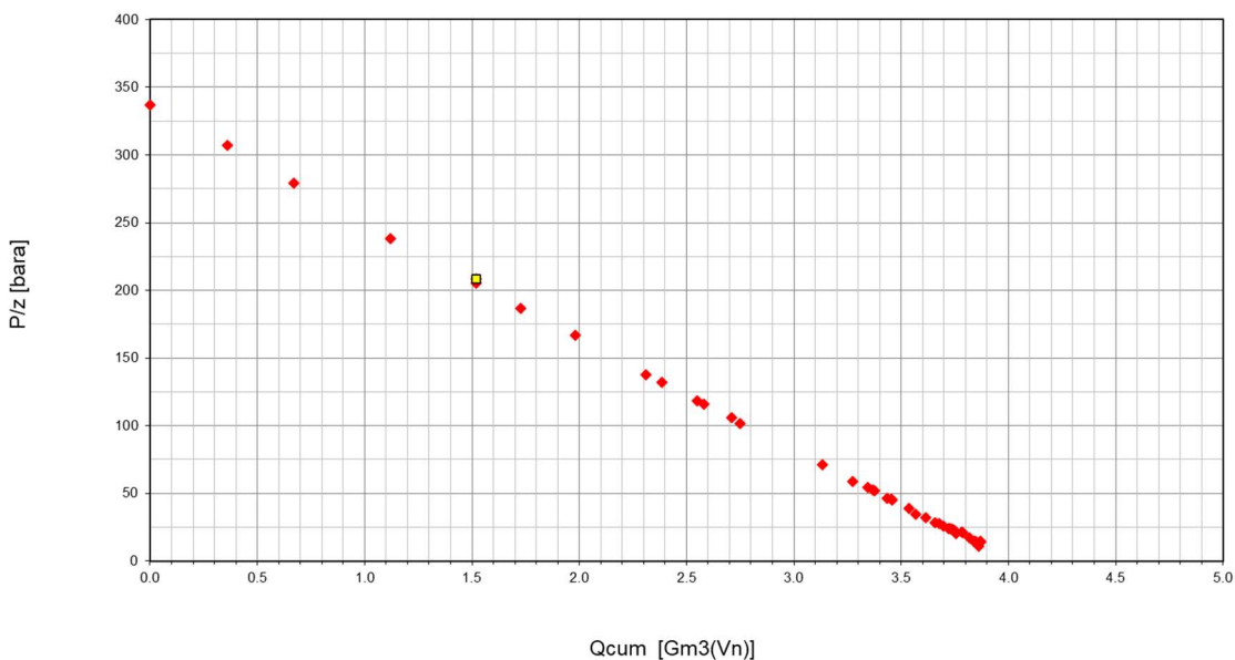
Figuur 10 p/z plot voor reservoir P15-9
