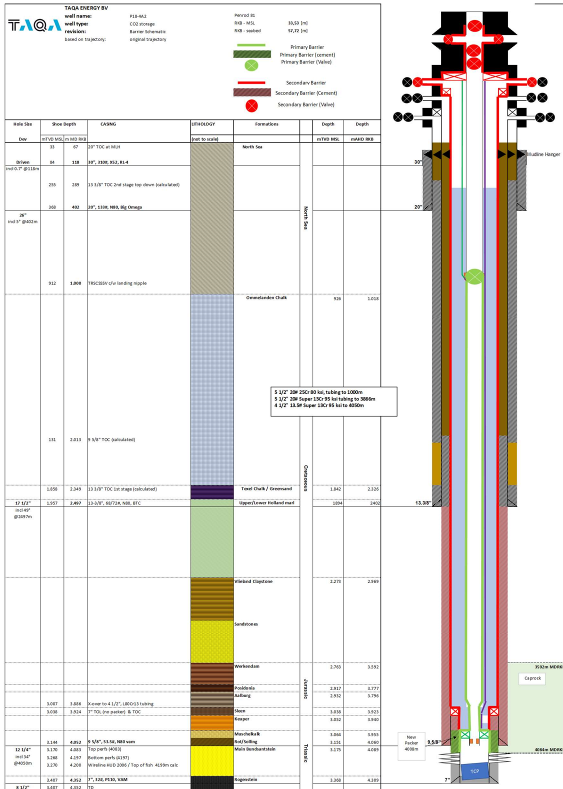
Figuur 28 Schema van de barrière van put P18-4A2 Groen is de primaire barrière en rood is de secundaire barrière.
