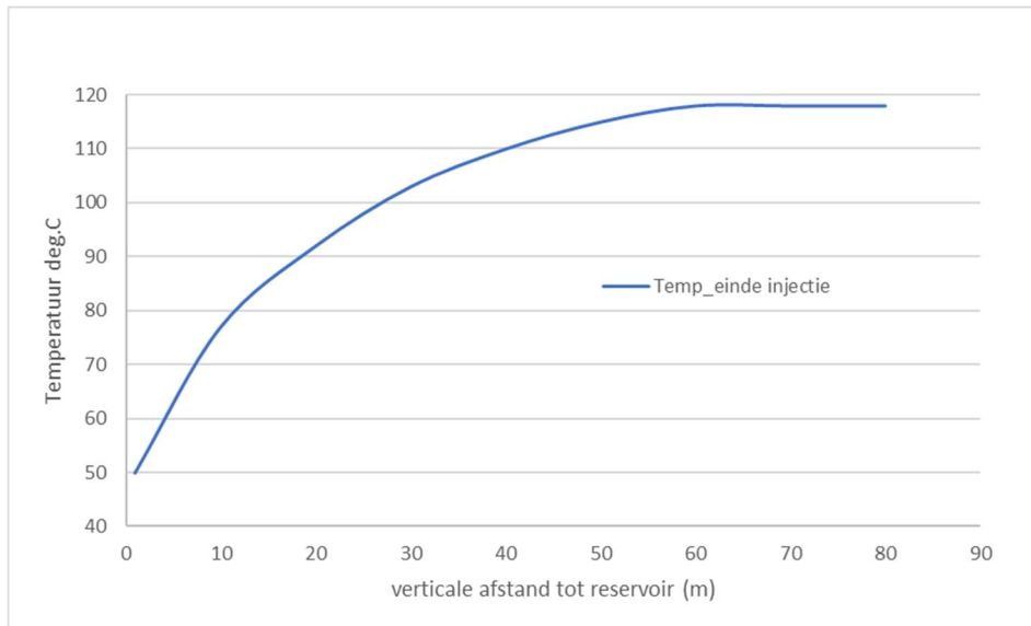
Figuur 24 Afkoeling van de overburden in P18-4A2 (zie SRA voor details).
