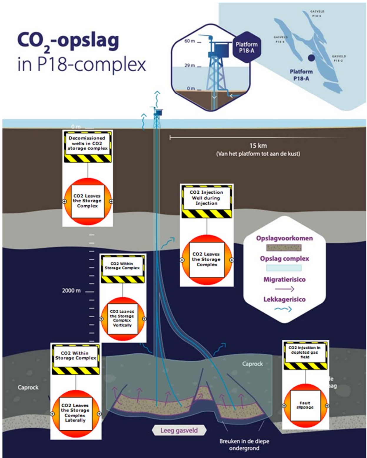
Figuur 10 Schematische weergave (niet op schaal) van ongewenste gebeurtenissen voor CO 2 -opslag in het opslagcomplex.
