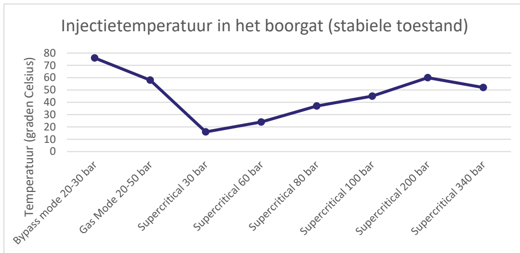
Figuur 40 Injectietemperatuur in het boorgat (stabiele toestand).
