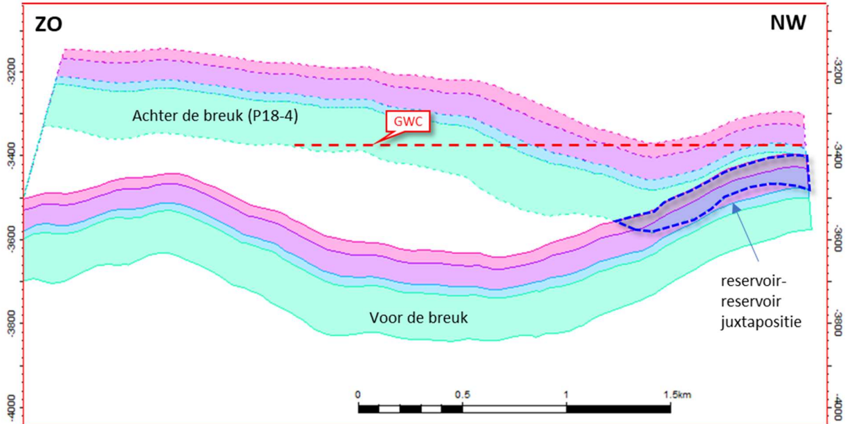
Figuur 6 Allan diagrammen van twee randbreuken van P18-4. Merk op dat de horizontale en verticale schaal van Figuren A en B verschillen.
