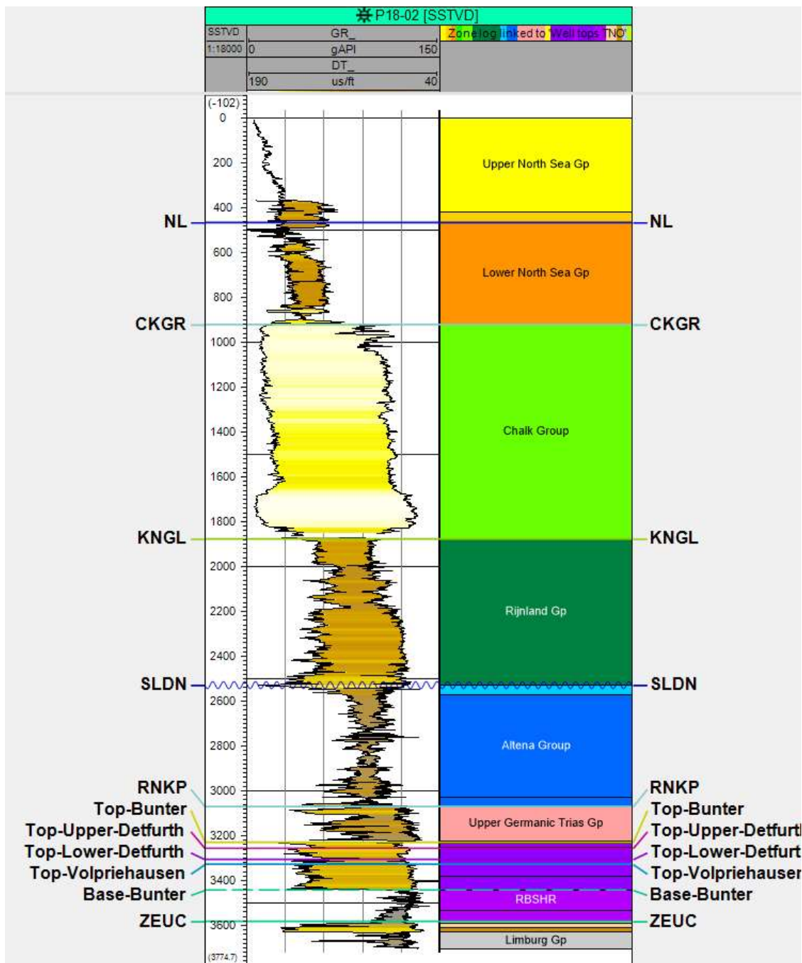
Figuur 13 Stratigrafie en Gamma Ray (GR) en Sonic (DT) eigenschappen van reservoir P18-2, met hoofdafdichting (Upper Germanic Trias Gp., Altena Gp.) en resterende overburden. Put P18-2 is een verticale put midden in de P18 velden en is representatief voor de stratigrafie in dit gebied.
