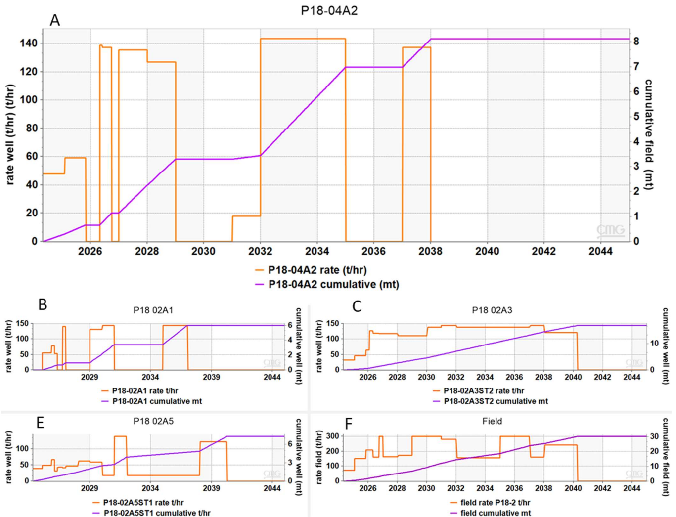
Figuur 17 Injectiesnelheden en cumulatieve opslag voor P18-4 (A). Het totale injectiedebiet voor P18-4 is geen continu plateau. Dit komt door de bijdrage van P18-2 (B t/m E). Het totale injectiedebiet van beide velden is 300 ton/uur (F).
