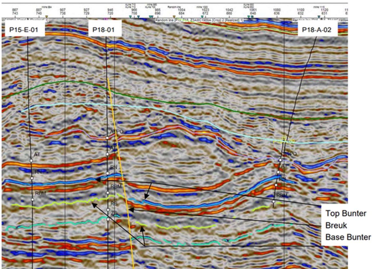
Figuur 7 Seismische weergave van breukzone tussen reservoir P18-4 en P15-9 (breuk P18-4 Noord)
