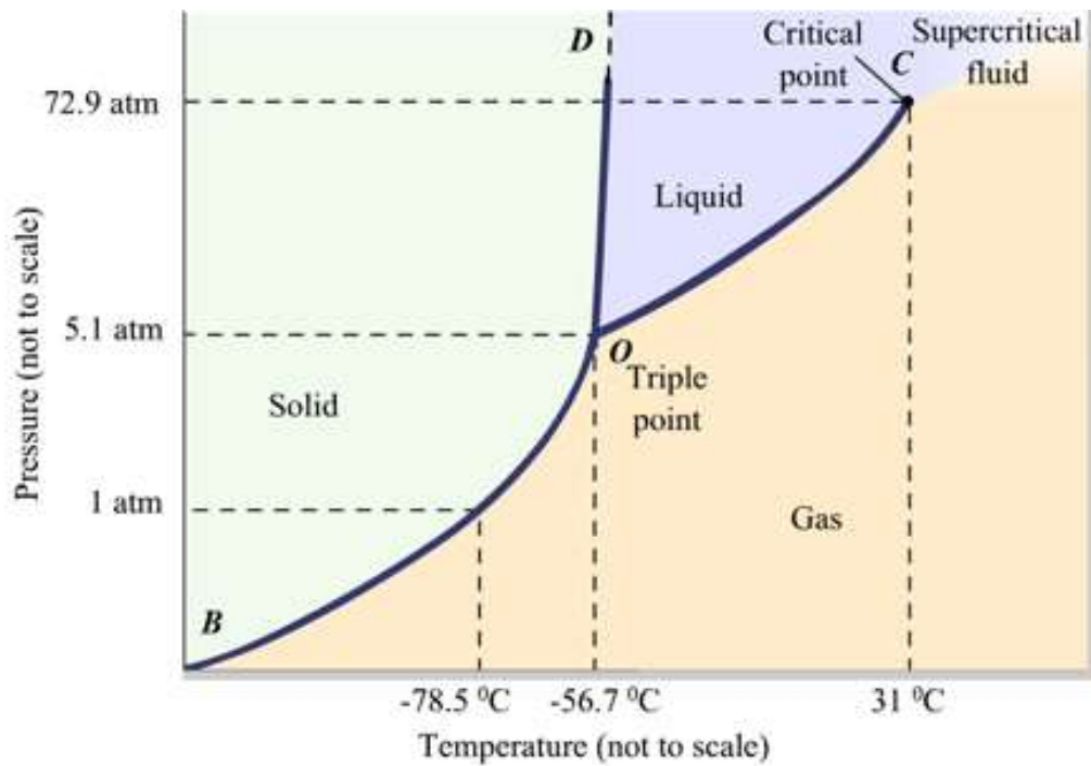
Figuur 29 Fasediagram CO 2 .
