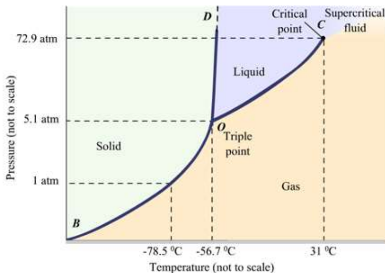
Figuur 18 Fase diagram voor zuivere CO 2 . (zie tekst voor uitleg)
