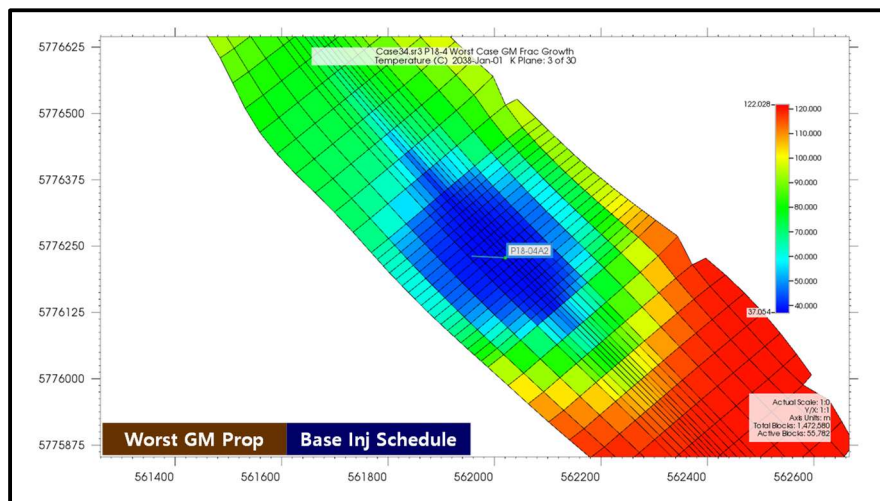
Figuur 23 Temperatuurprofiel met thermische scheurvorming bij put P18-4A2 (resultaten afkomstig uit de stresstest).
