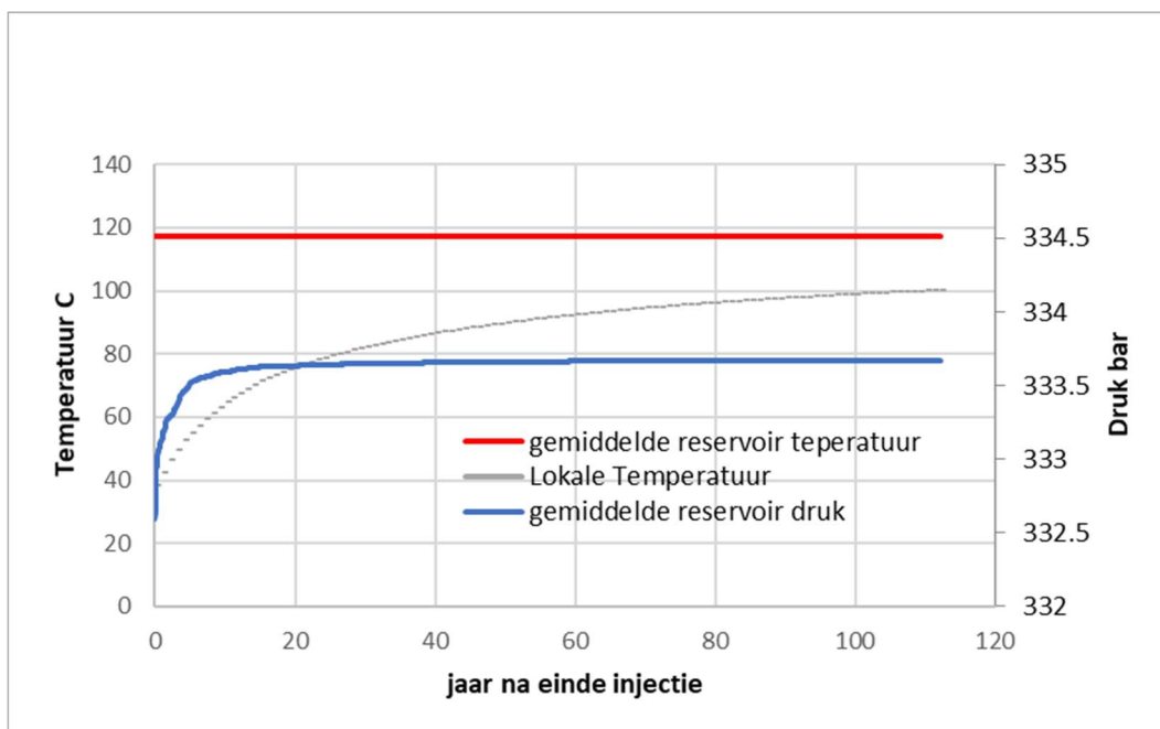
Figuur 22 Drukverandering (gemiddelde reservoir druk in blauw) in het reservoir als gevolg van opwarming na injectie (gemiddelde reservoir teperatuur in rood). De grijs gestippelde lijn geeft de lokale temperatuuropbouw weer na insluiten van P18-4A2 aan het eind van de injectie.
