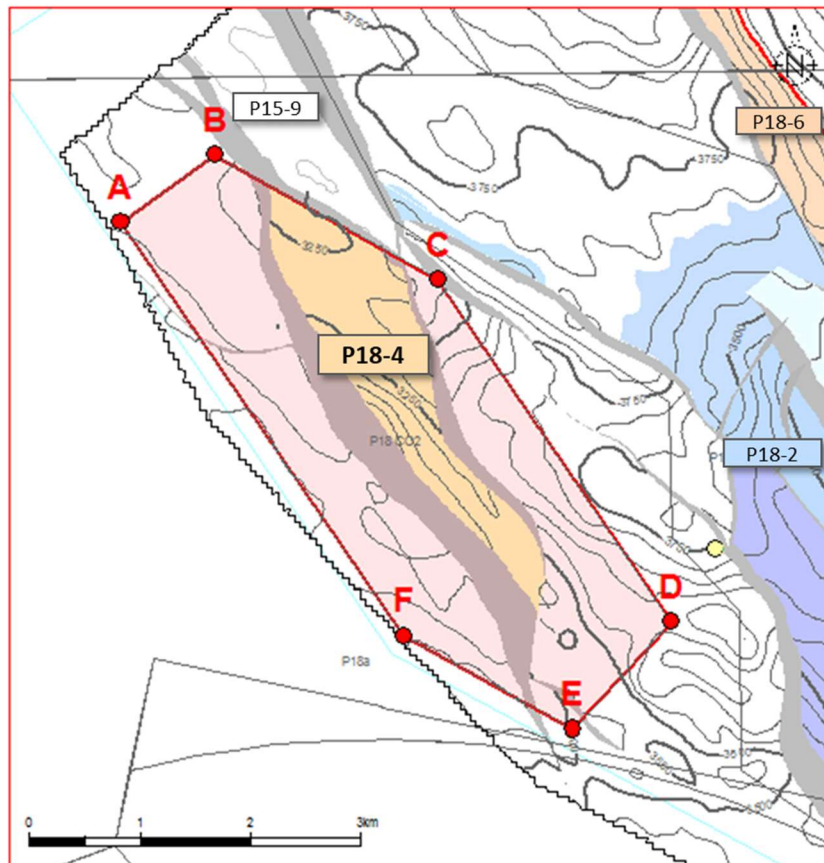
Figuur 2 Contour van het Opslagcomplex P18-4, gedefinieerd door hoekpunten A t/m F. De contour is hier weergegeven op een kaart van de bovengrens van de Hoofd-Germaanse Bontzandsteen Subgroep (diepte in meters onder zeeniveau), ook de bovengrens van reservoir P18-4. Zie Deel I, Paragraaf 5.3 voor beschrijving van de omvang van het vergunningsgebied.
