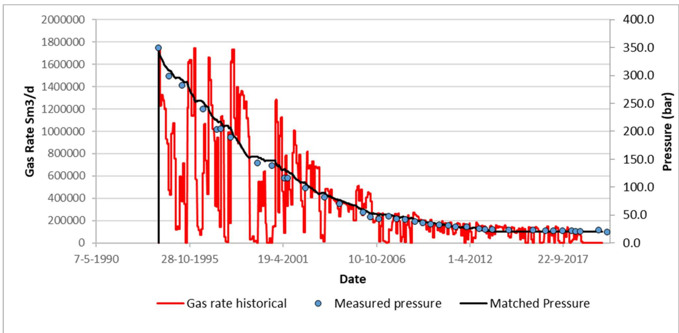
Figuur 16 Kalibratie van het dynamisch model: de gesimuleerde putdrukken (zwarte lijn) komen overeen met de gemeten drukken. Gas rates worden weergegeven (rode lijn).
