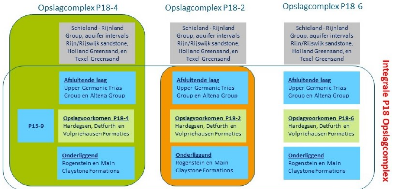
Figuur 2 Overzicht van het Integrale P18-opslagcomplex.
