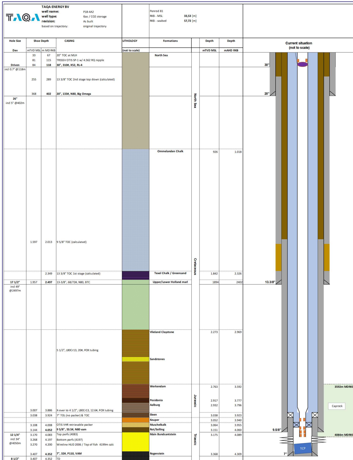
Figuur 25 Diagram huidige status put P18-4A2.
