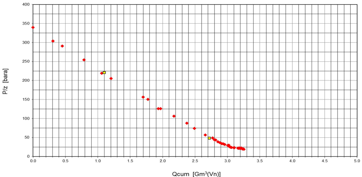
Figuur 11 p/z plot voor reservoir P18-4A2
