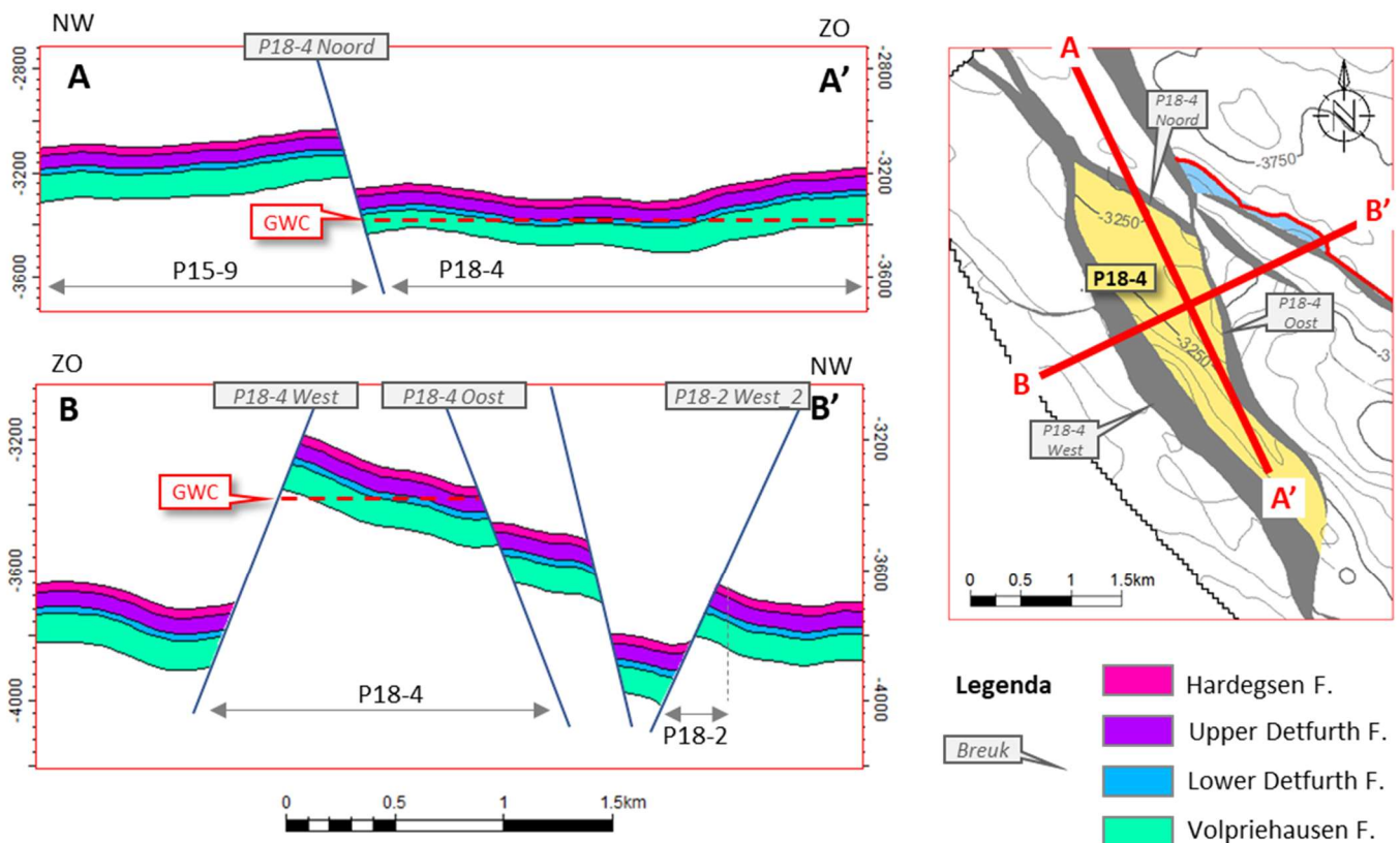
Figuur 5 Twee dwarsdoorsnedes door het P18-4 reservoir. Aangegeven zijn de vier formaties. Het verzet langs de randbreuken is zodanig dat de reservoirs zijdelings worden begrensd door afdichtend gesteente in de afsluitende laag. Het verzet overstijgt echter niet de dikte van de afsluitende laag, zodat langs de hele structuur reservoir lateraal tegen primaire afsluitende laag is geplaatst.
