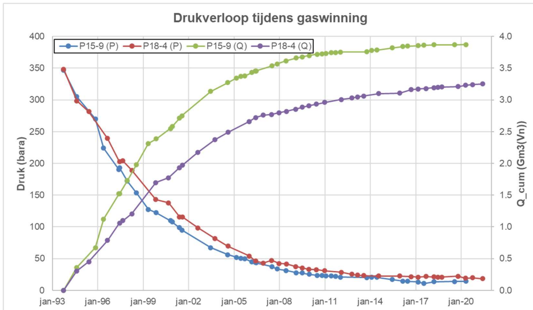
Figuur 9 Overzicht productie en reservoir voor P18-4 en P15-9
