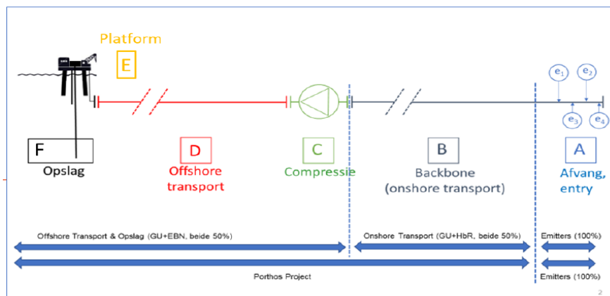
Figuur 8 Het Porthos Systeem.
