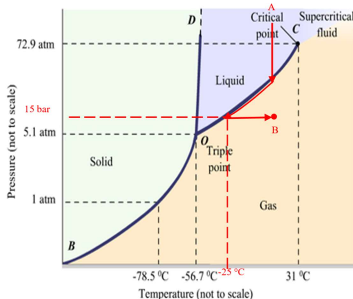
Figuur 19 Illustratie van afkoeling beschreven als voorbeeld in de tekst.
