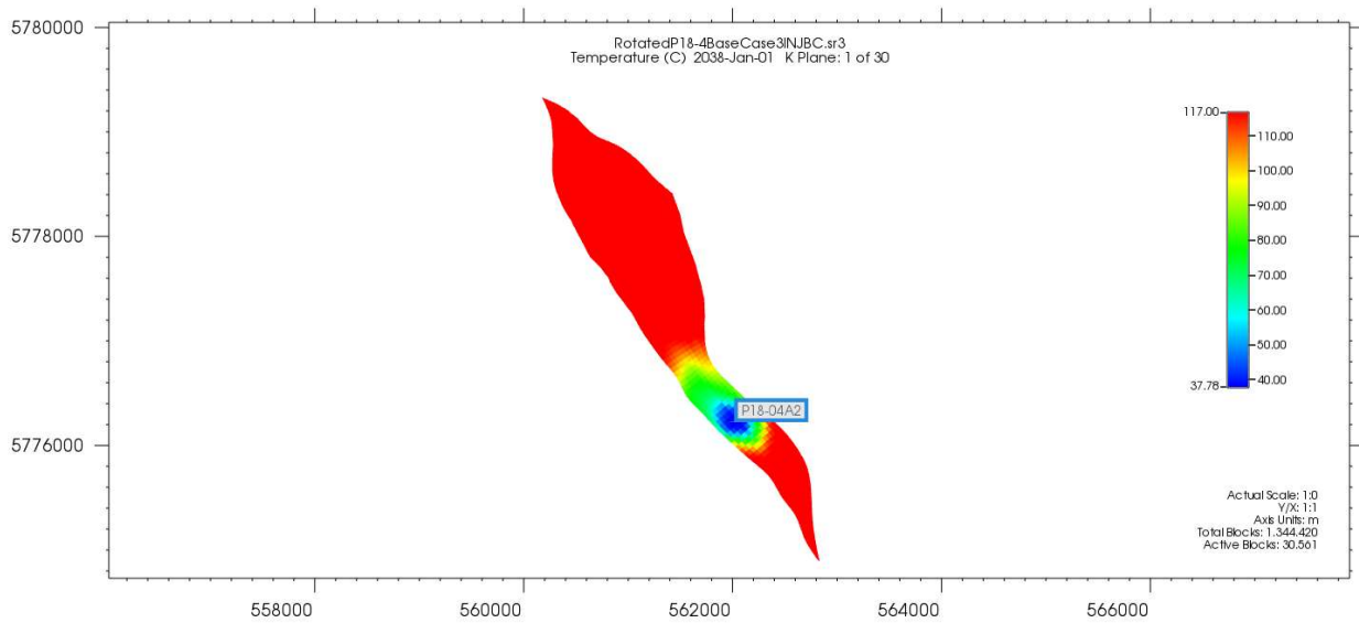
Figuur 21 Temperatuurprofiel in het reservoir aan het eind van de injectie.
