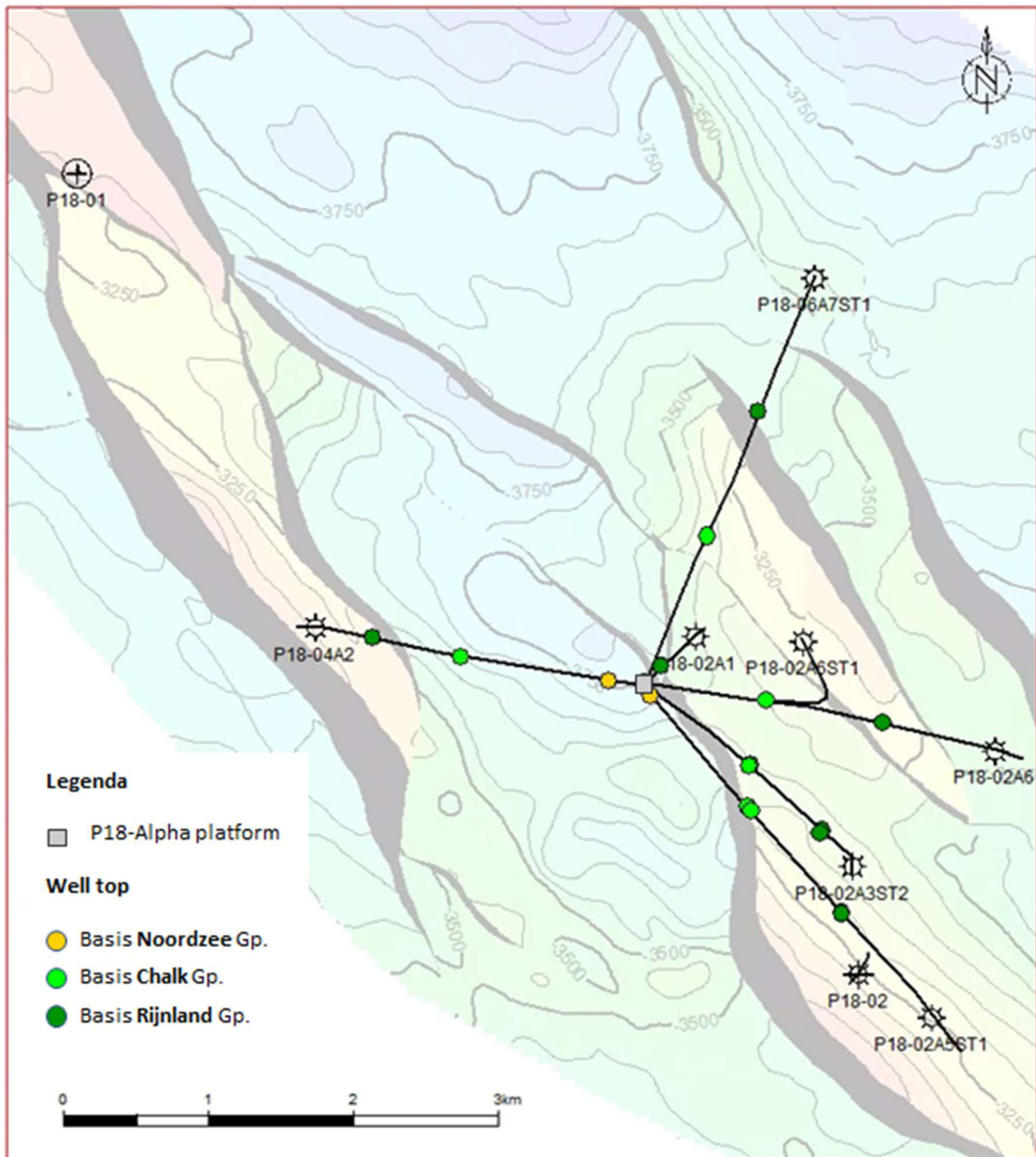
Figuur 14 Overzichtskaart het boorgattraject van P18-4A2 in het P18-4 reservoir met putsymbool en -naam weergegeven ter hoogte van het snijpunt met de top van het Bunter-reservoir (voor het overzicht zijn ook de producerende putten in P18-2 en P18-6 weergegeven).
