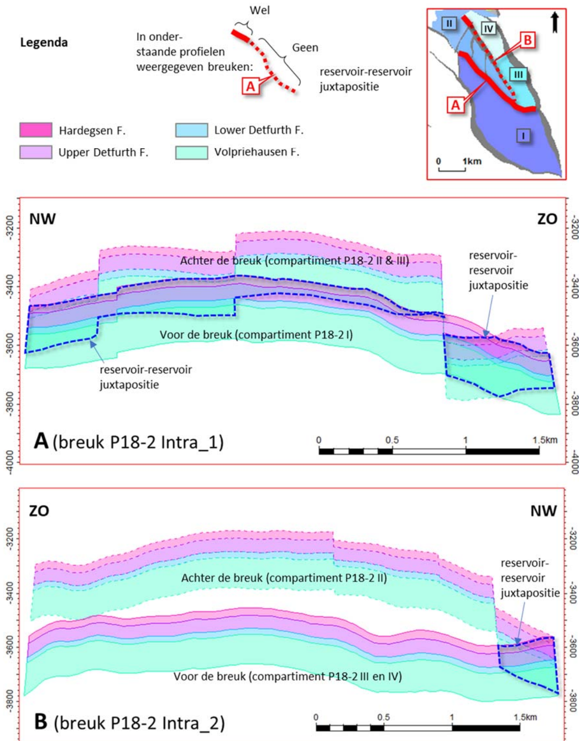
Figuur 16 Allan diagrammen voor twee interne breuken in het P18-2-veld. Aangegeven zijn de vier reservoirniveau's die in het statische reservoirmodel zijn opgenomen en het gebied waarin eventuele reservoir-reservoir juxtapositie plaatsvindt.
