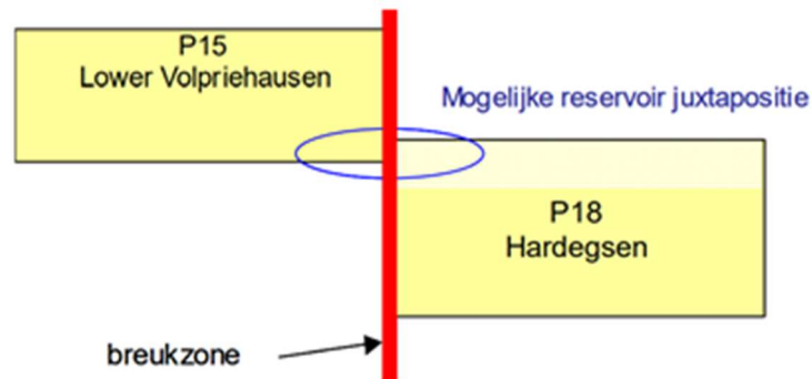
Figuur 8 Schematische weergave van de mogelijke reservoir juxtapositie tussen reservoir P18-4 (Hardegens, lichtgeel) en P15-9, aan de noordwestzijde (Lower Volpriehausen, donkergeel)
