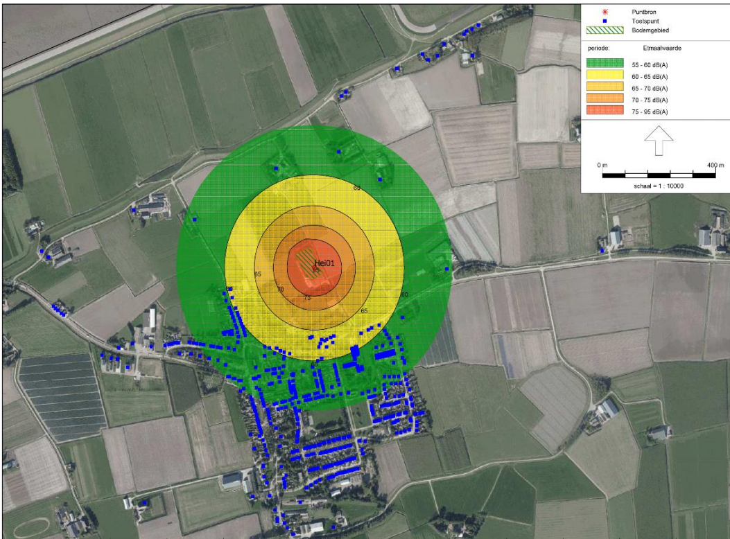
Figuur 13-10 Geluidscontouren heiwerkzaamheden in de dagperiode Locatie 1
