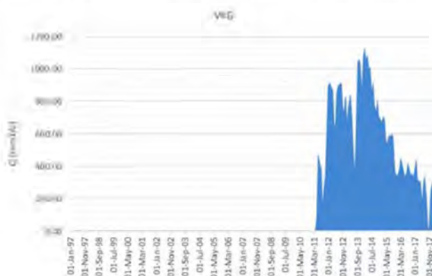
Figuur 2-5: Vinkega productiegeschiedenis. De twee Vinkega putten produceren gezamenlijk (commingled) uit Vleiland en Rotliegend.
