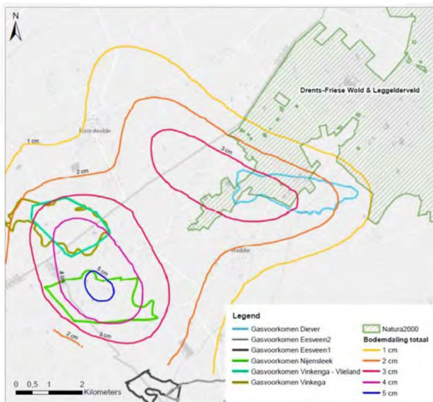
Figuur 18-5 Samengestelde bodemdaling totaal in cm bij einde productie
