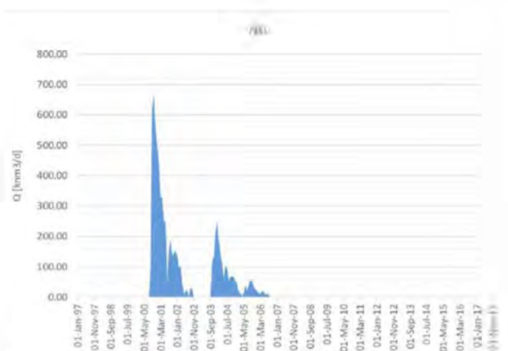
Figuur 2-3: Nijensleek productiegeschiedenis. De productie is beëindigd door uitwatering bij 23 bar, bij een initiële druk van 221 bar.
