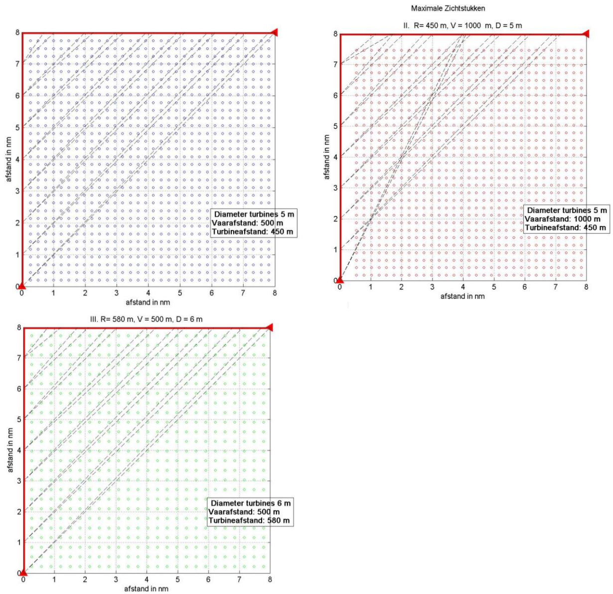
Figuur 3-15 Linksboven: Opstelling windturbines in vierkant evenwijdig aan vaarlinks, vaarafstand 500 m , rechtsboven: opstelling windturbines in vierkant evenwijdig aan vaarlinks, vaarafstand 1000 m linksonder: opstelling windturbines in vierkant evenwijdig aan vaarlinks, afstand tussen turbines 580 m en vaarafstand 500 m
