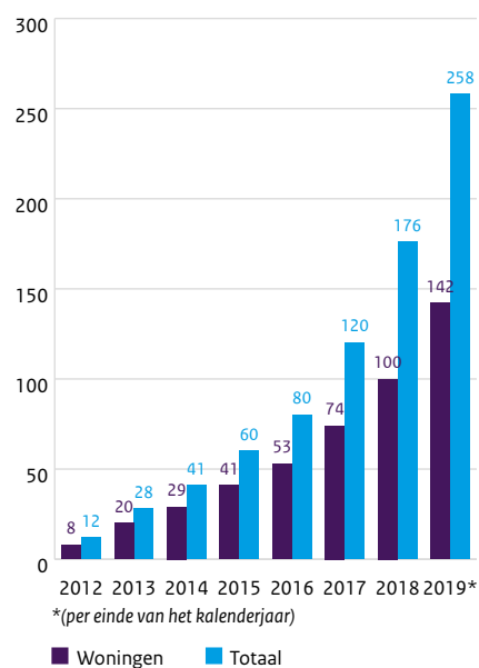
Opgesteld vermogen in de regio (in MWp)
