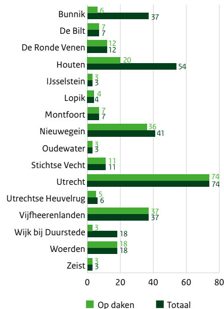
Vermogen van SDE+ projecten die nog in de pijplijn zitten (in MWp)
