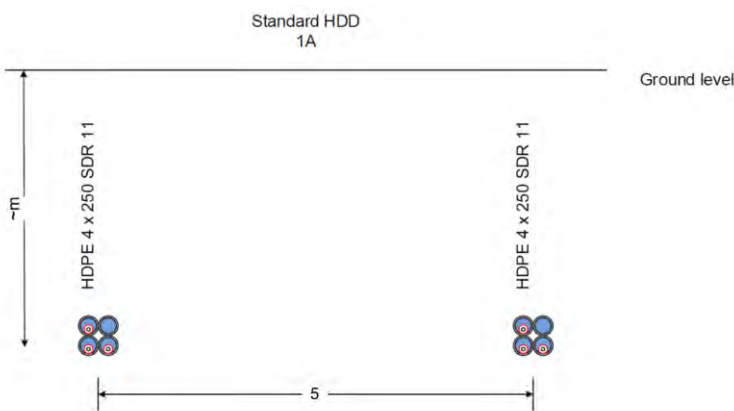
Afbeelding 2.3 Doorsnede gestuurde boring (twee circuits)
