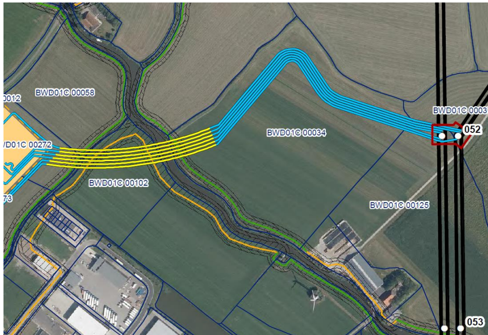
Figuur 6 Voorgenomen kabeltracé van 110kV hoogspanningsstation naar opstijlpunten
