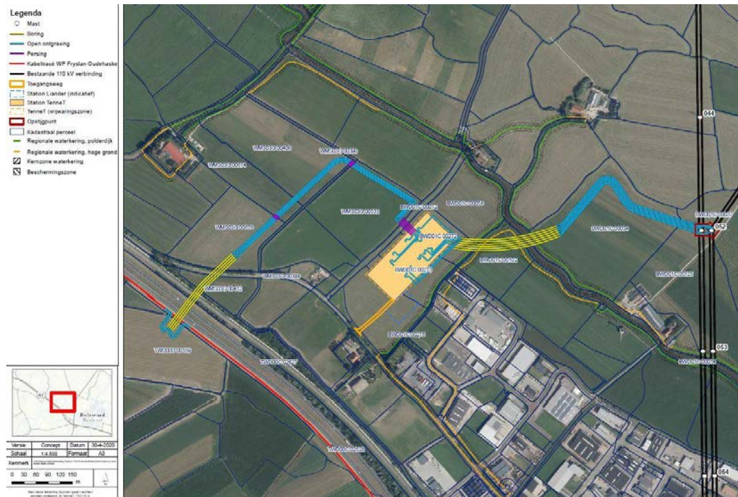
Figuur 1 Overzicht station Bolsward 110 en kabeltracés
