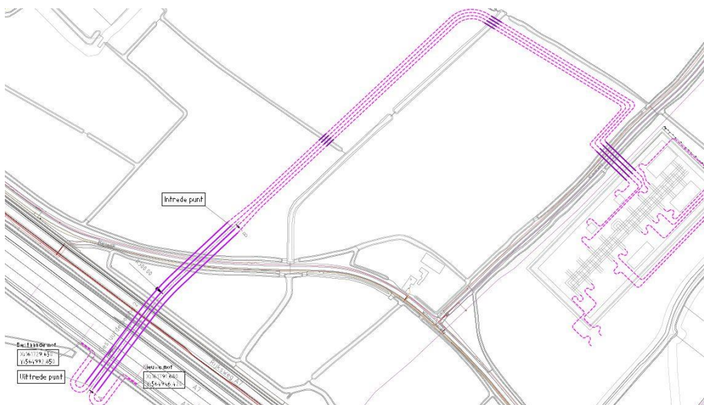
Figuur 4 Voorgenomen kabeltracé van A7 tot 110kV hoogspanningsstation
