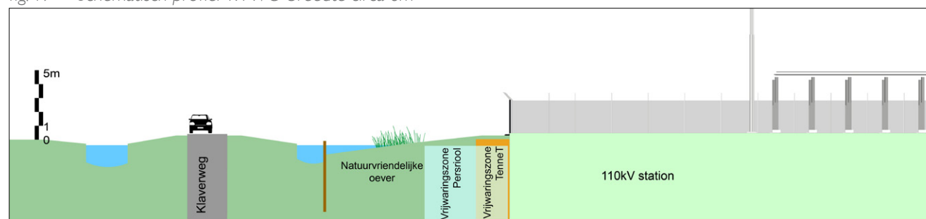
fig. 18 Schematisch profiel 2: NVO breedte circa 3m
