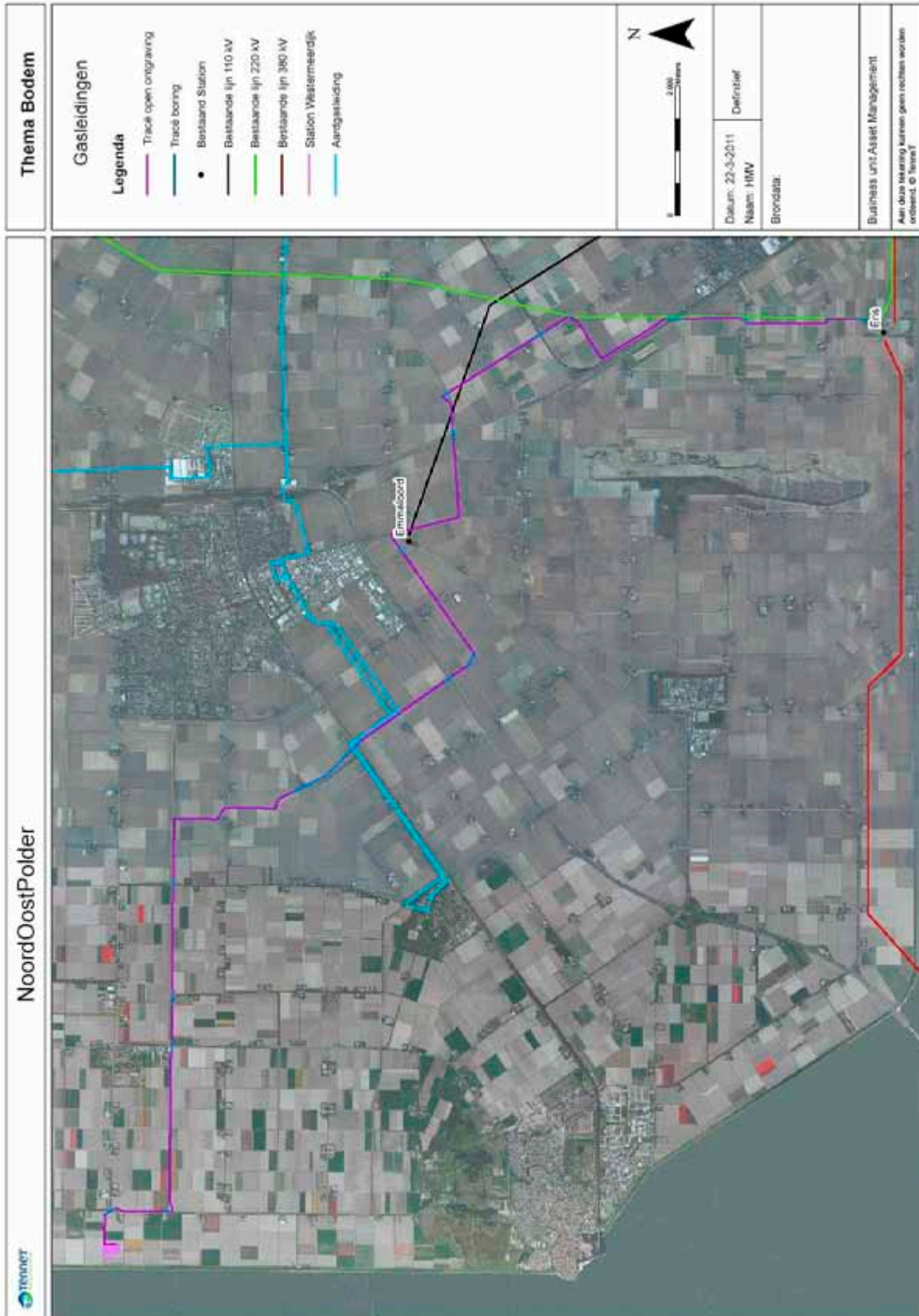
Figuur 15 Leidingen
