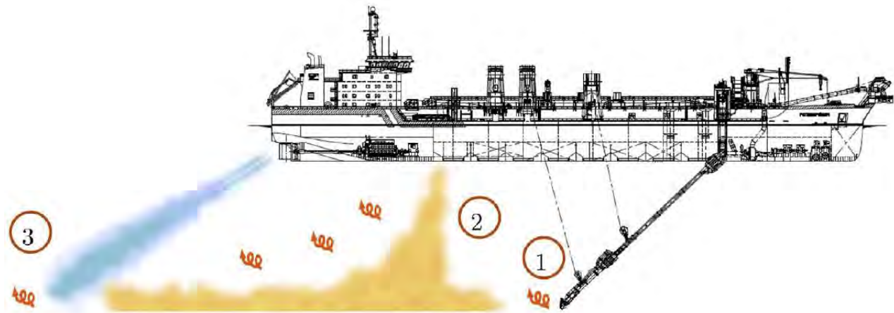
Figuur 6: Schematische weergave van de oorzaken van het in suspensie komen van slib tijdens baggerwerkzaamheden met een sleepopperzuiger.
