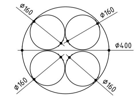
Boring bestaat uit 4 mantelbuizen HDPE Ø160mm, omhullende diameter bedraagt circa 400mm
