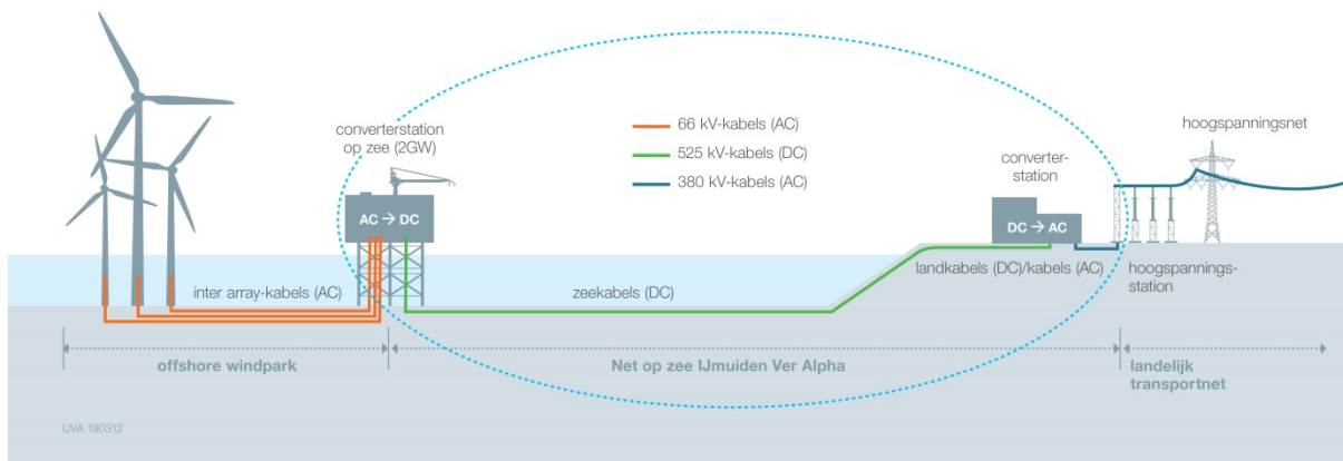
Figuur 1 Dwarsdoorsnede project
