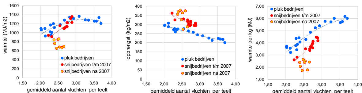
Figuur 12, 13 en 14: gemiddeld aantal vluchten per teelt en het energieverbruik voor warmte per m 2 , de opbrengst per m 2 en de warmte per kg.
