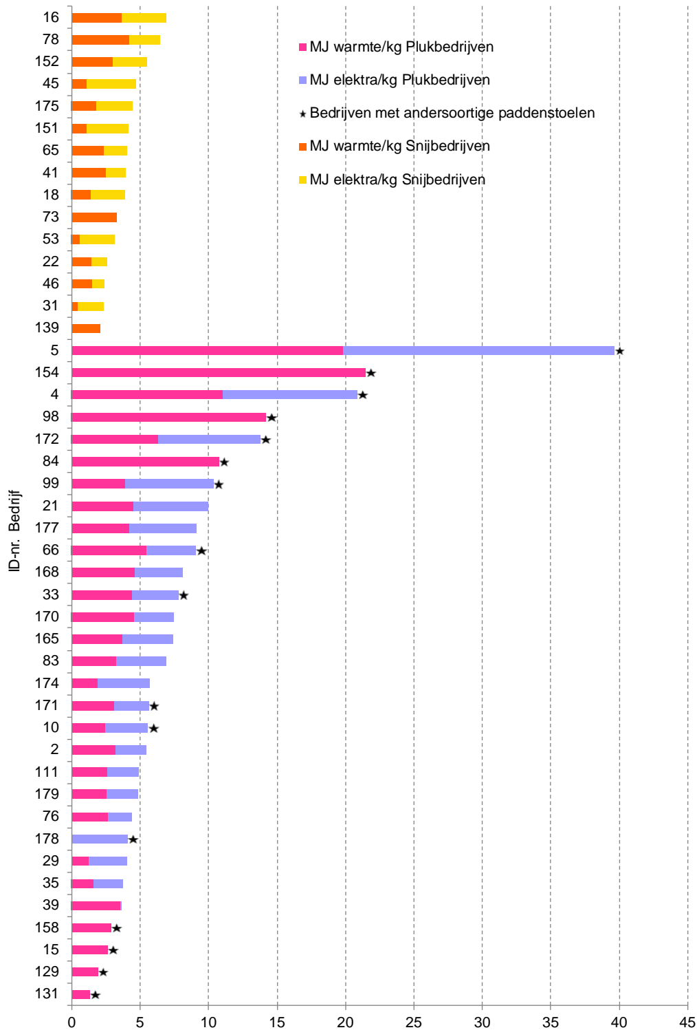
Figuur 20: Fossiel Energieverbruik per kg paddenstoelen (MJ/kg)
