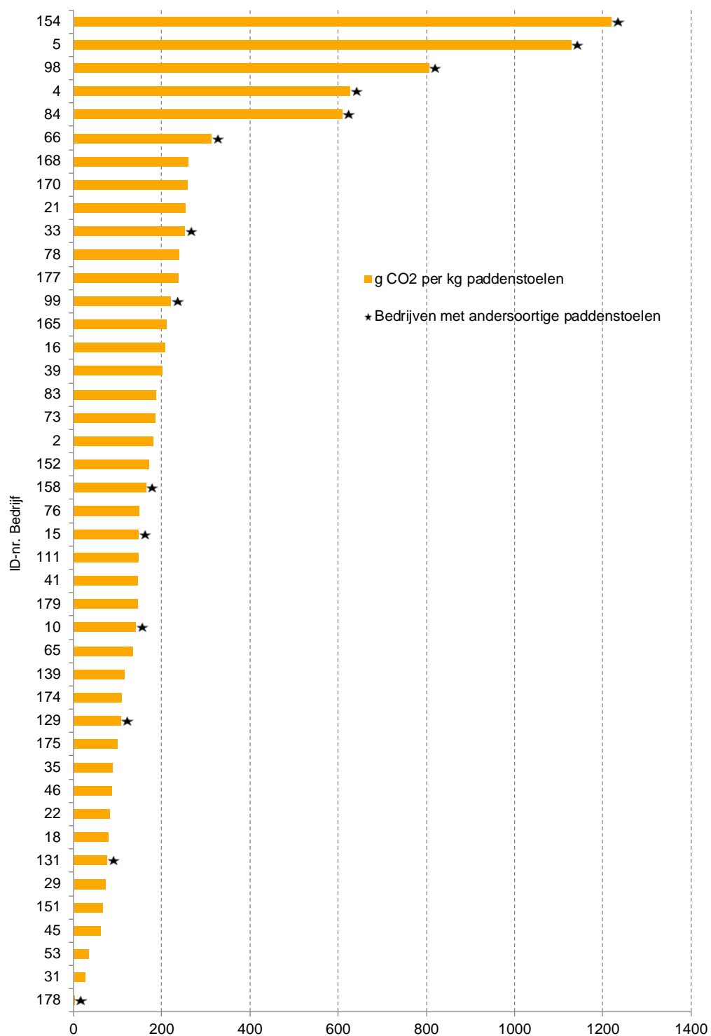
Figuur 19: CO 2 uitstoot/ kg paddenstoelen(g/kg) voor verwarming
