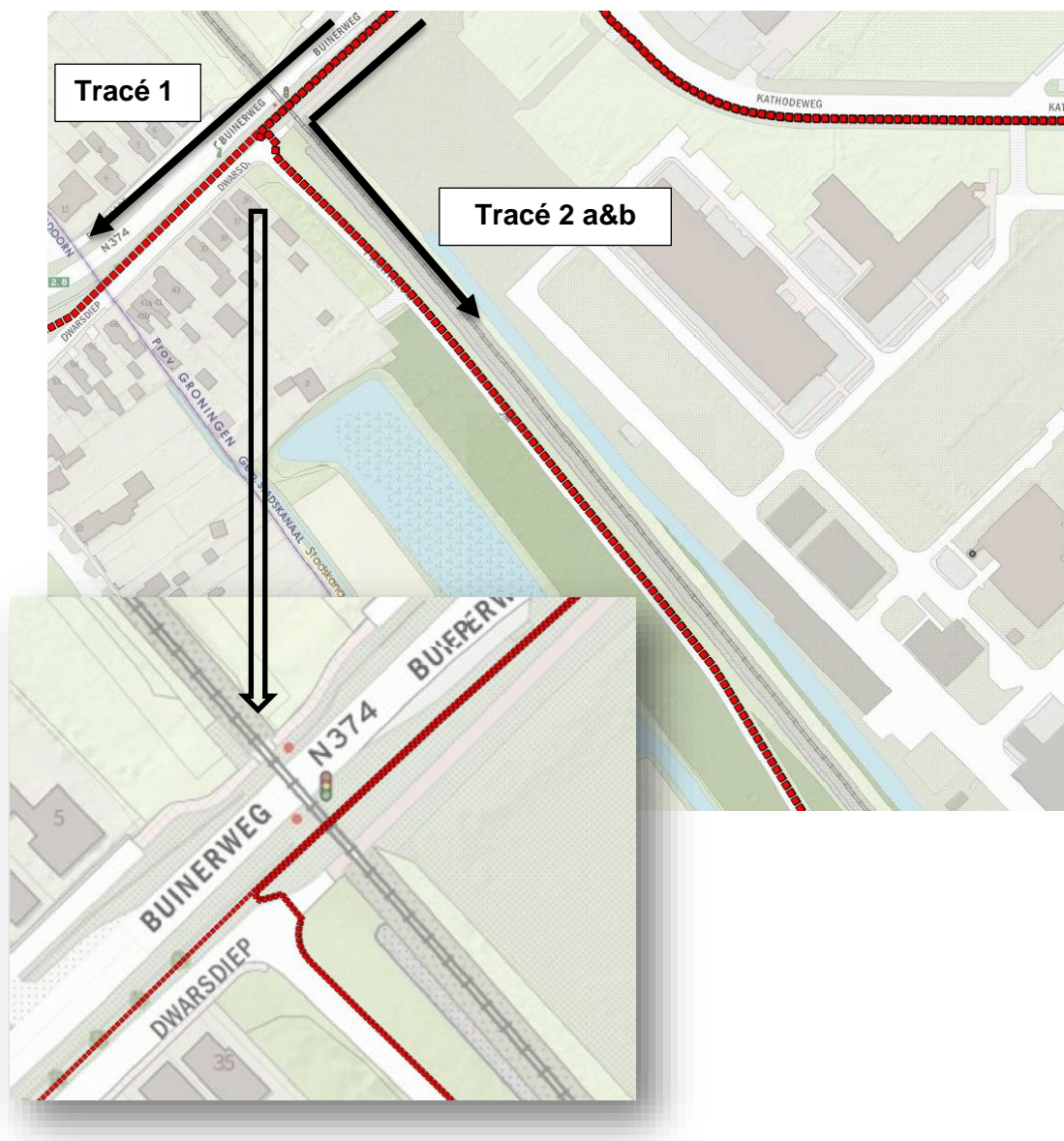
Figuur 2.4 Detail locatie C: kruising middels gestuurde boring + parallel op afstand van circa 10 meter tot het spoor over een lengte van circa 200 meter
