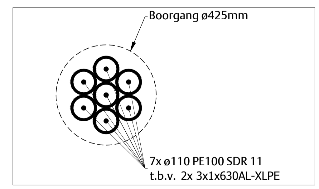
Doorsnede schaal 1 : 10
