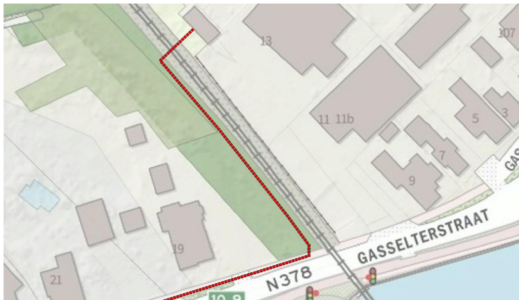
Figuur 2.3 Detail locatie B: kruising middels persing + parallel op afstand van circa 3 meter tot het spoor over een lengte van circa 70 meter
