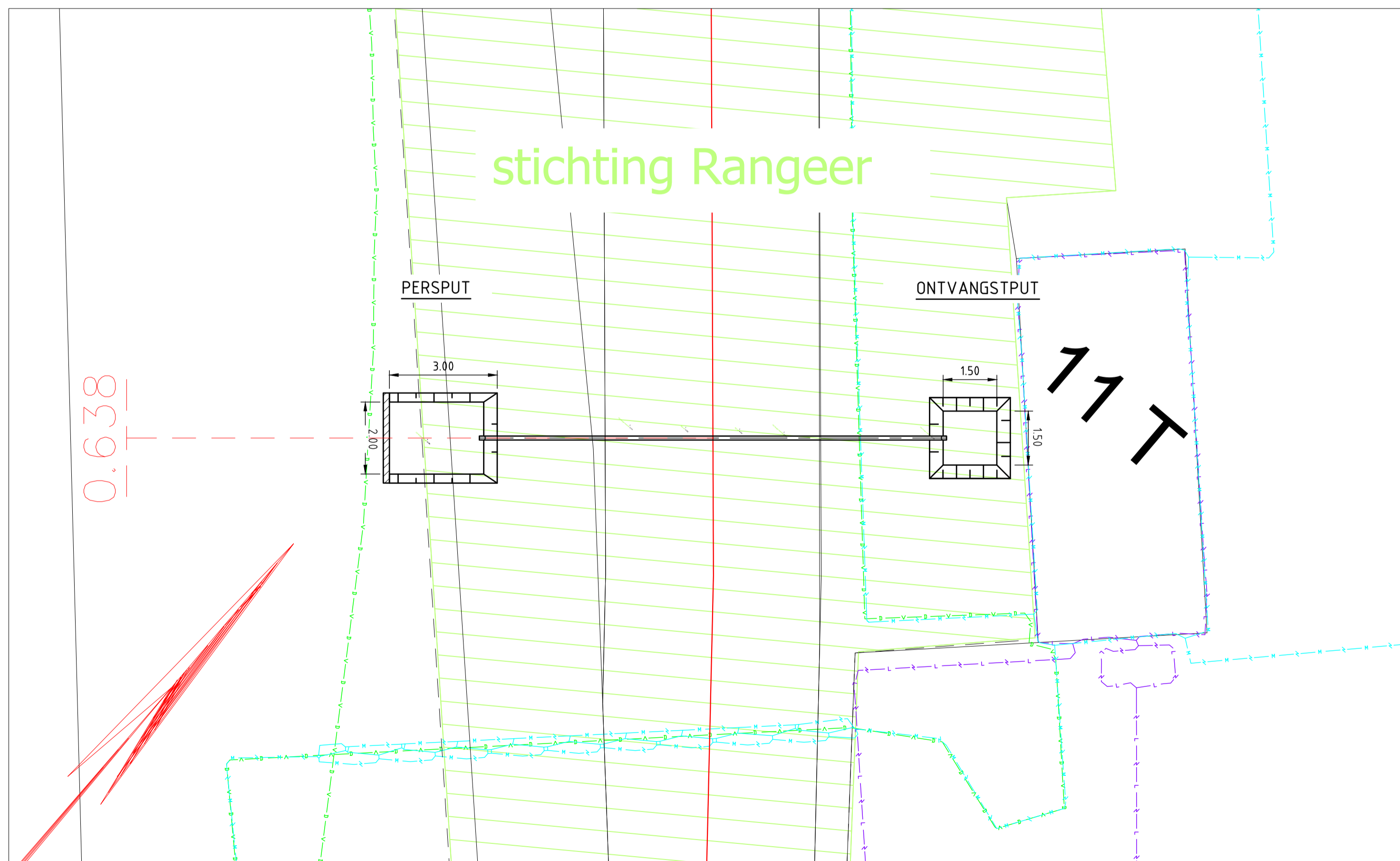
BOVENAANZICHT schaal 1 : 10
