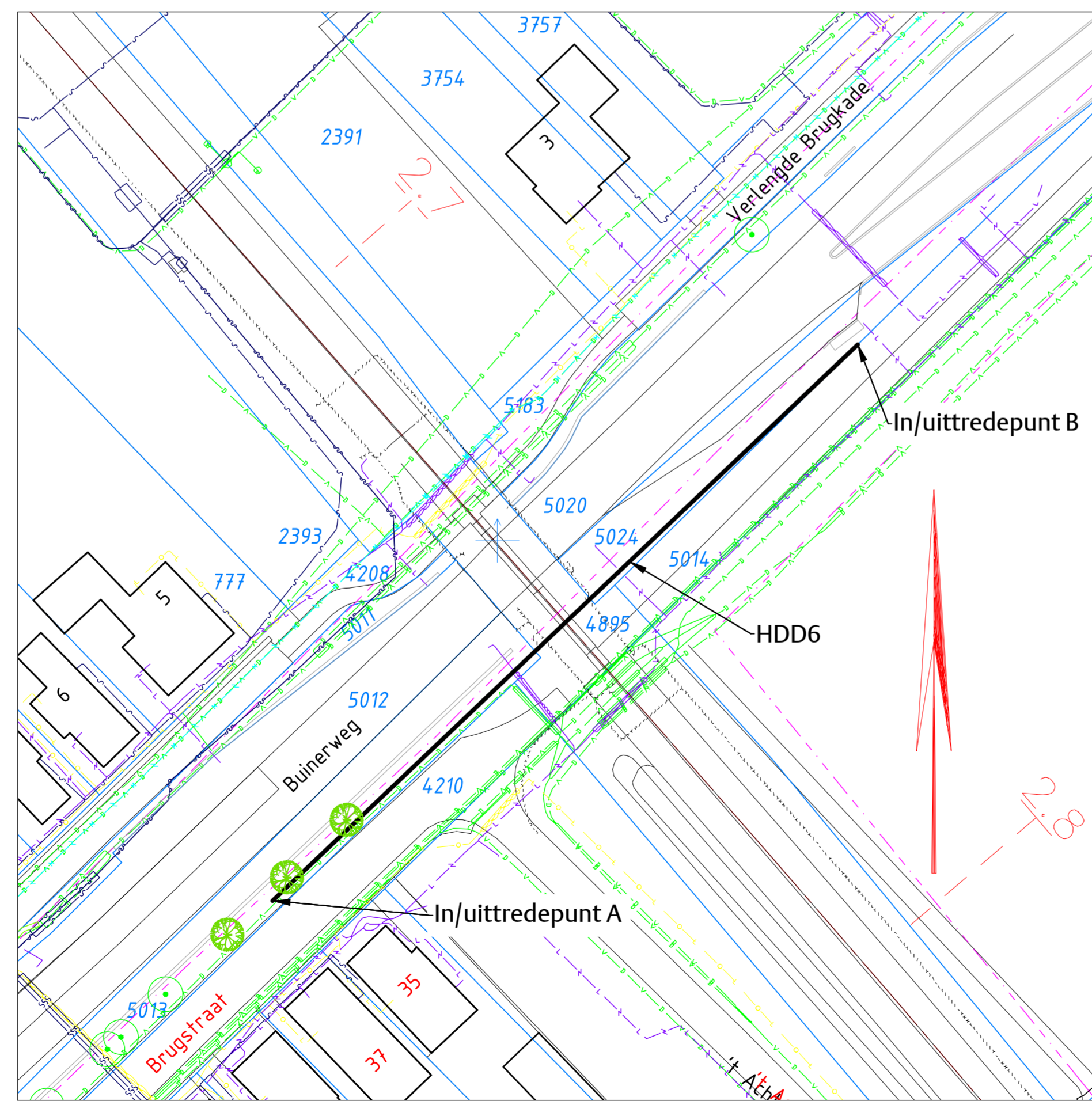
SITPLAN met klik schaal 1 : 100
