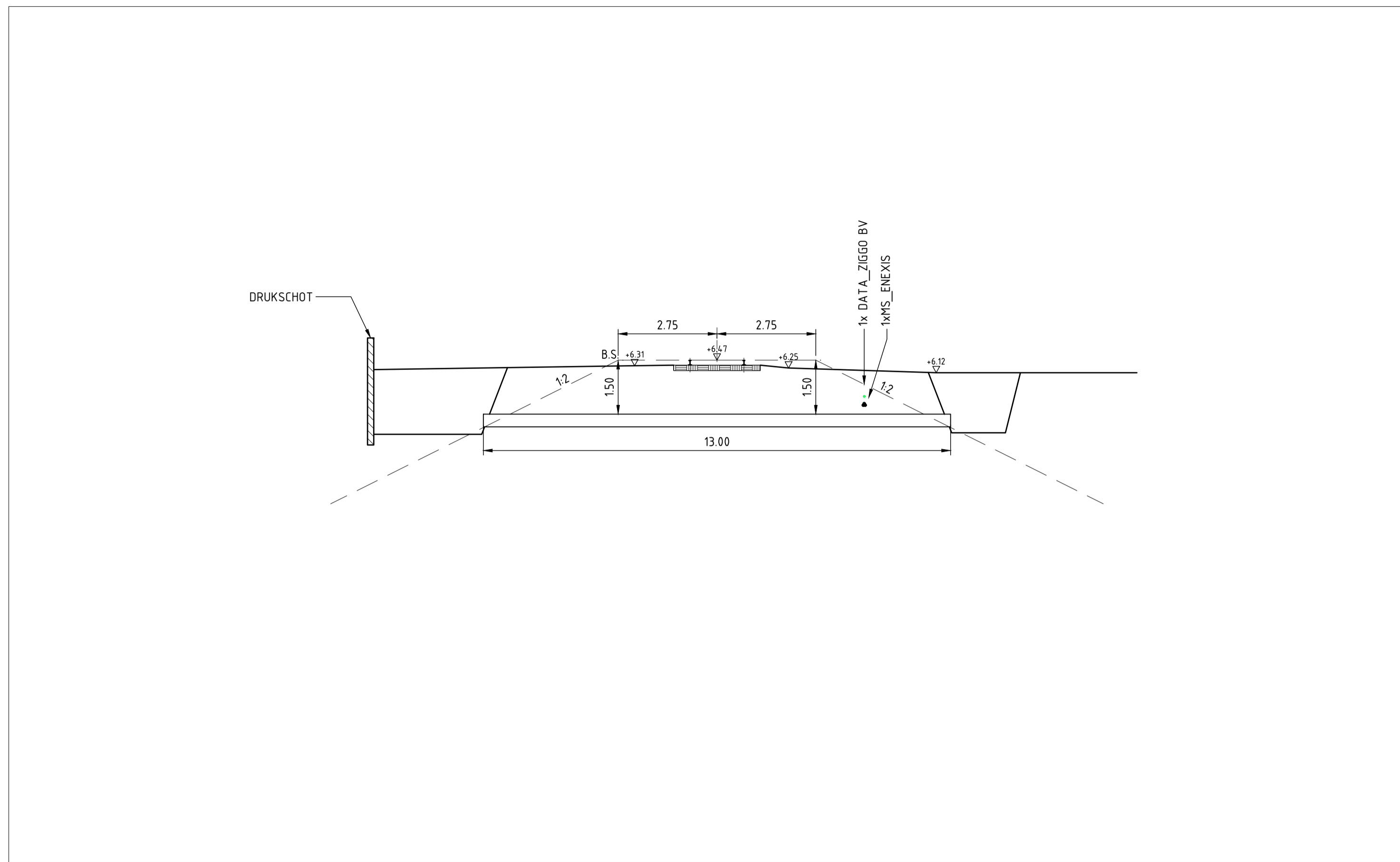
LANGSDOORSNEDE schaal 1 : 100
