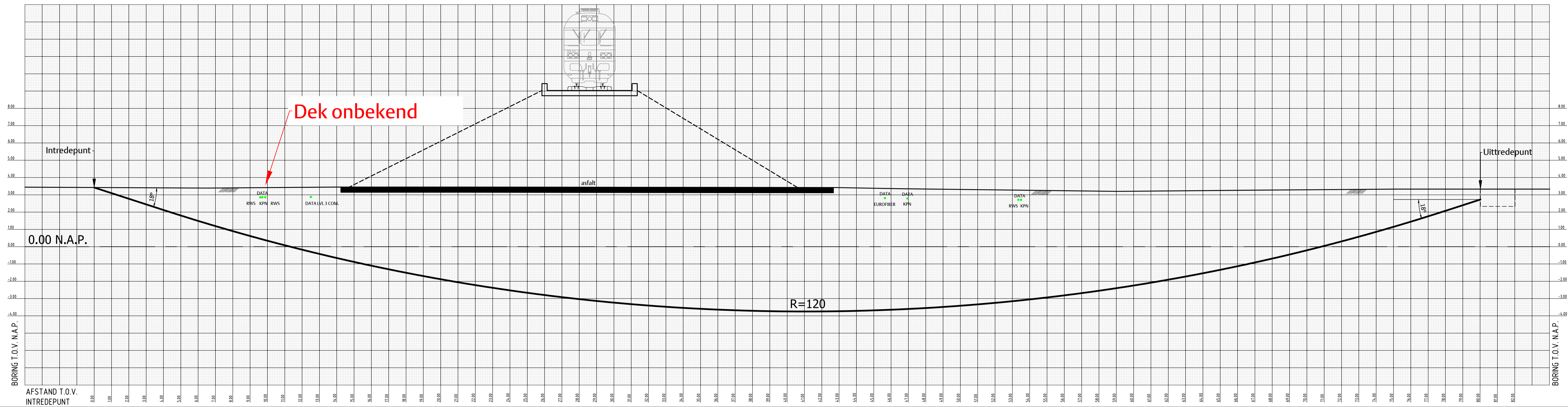
DIEPTEPROFIEL schaal 1 : 100
