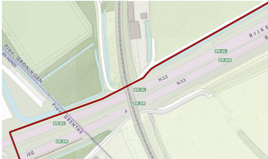
Figuur 2.2 Detail locatie A: kruising parallel aan N33 onder het bestaande spoorviaduct middels boring
