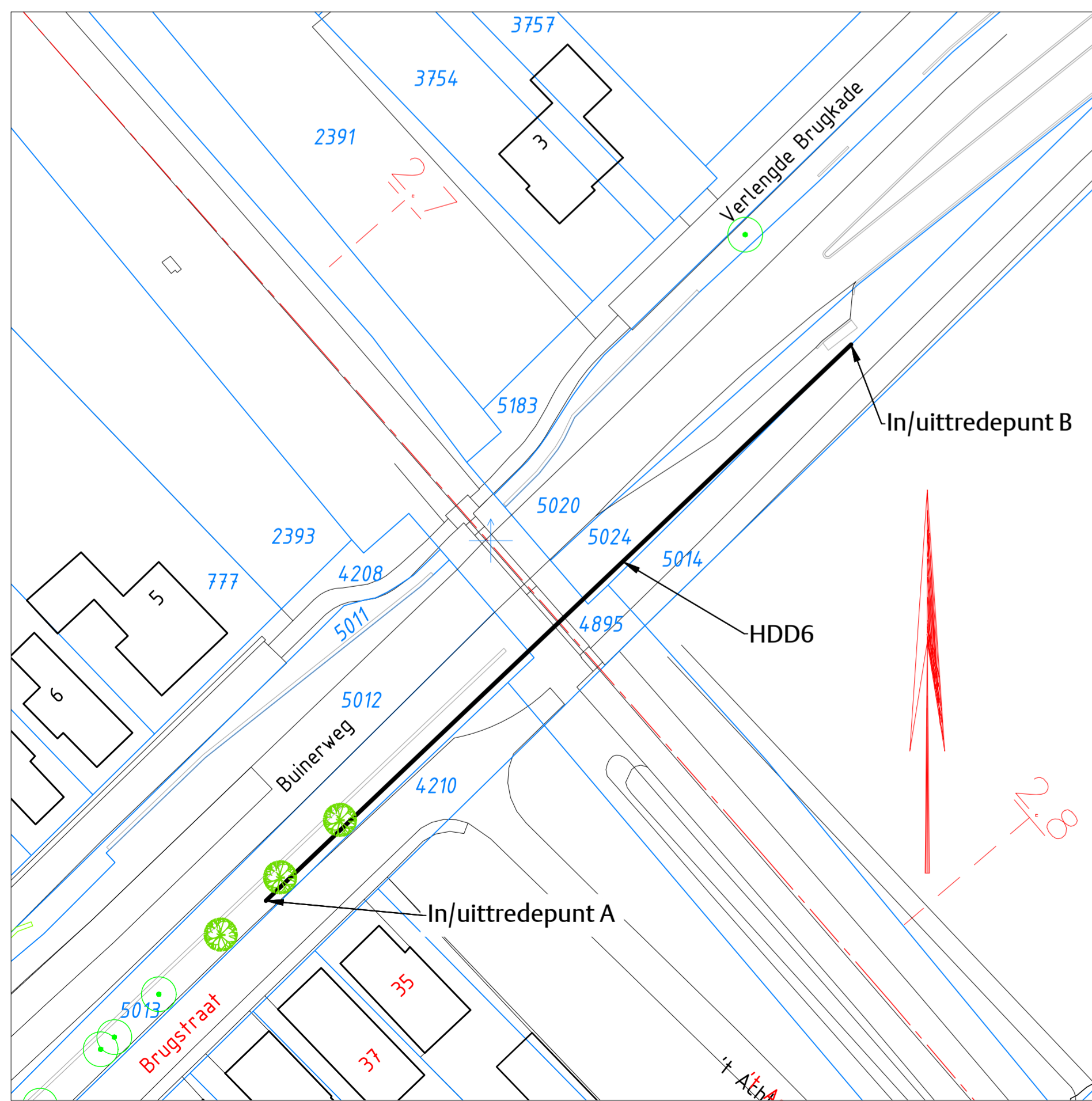
SITPLAN schaal 1 : 100
