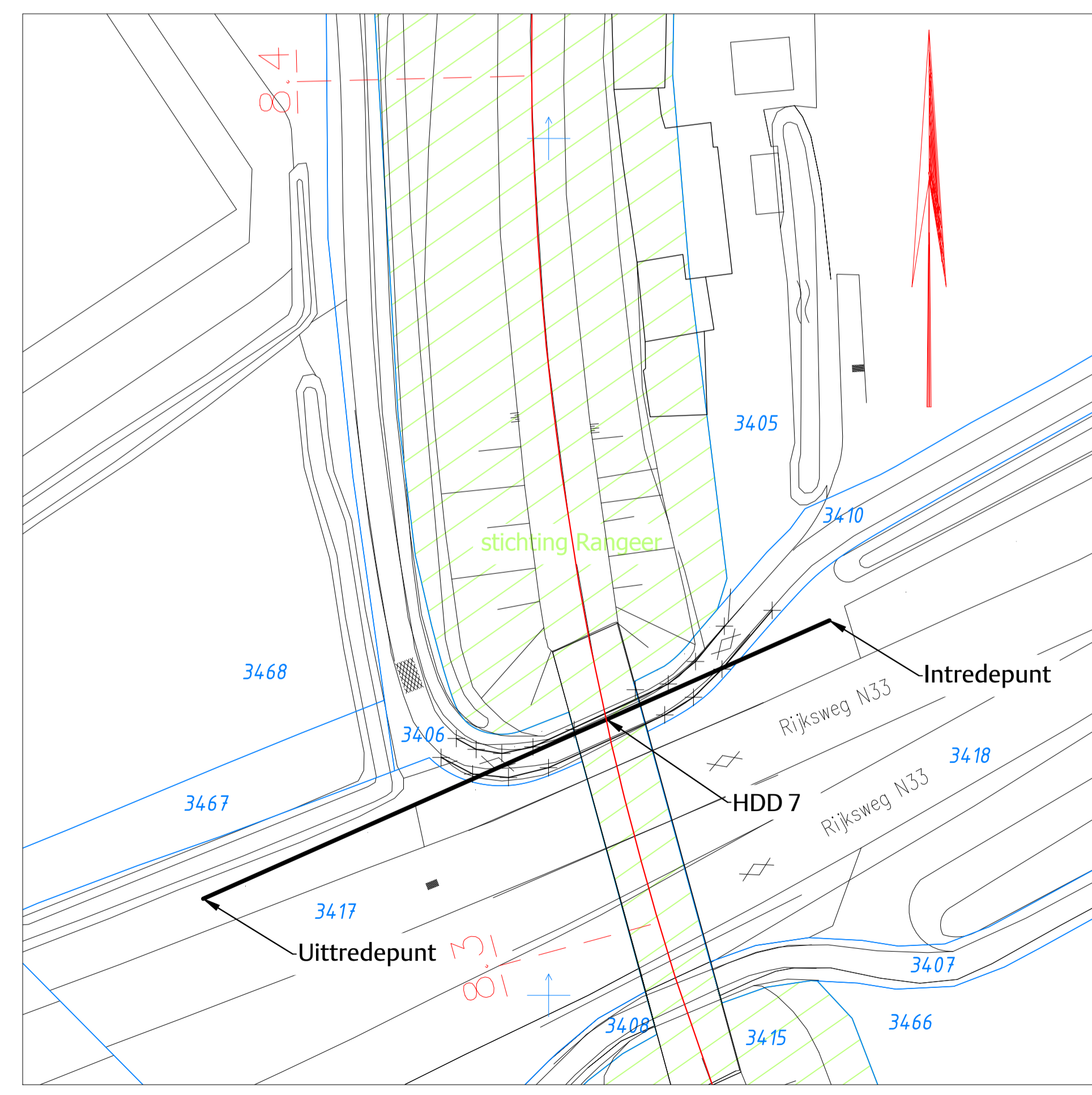
SITUATIE schaal 1 : 500
