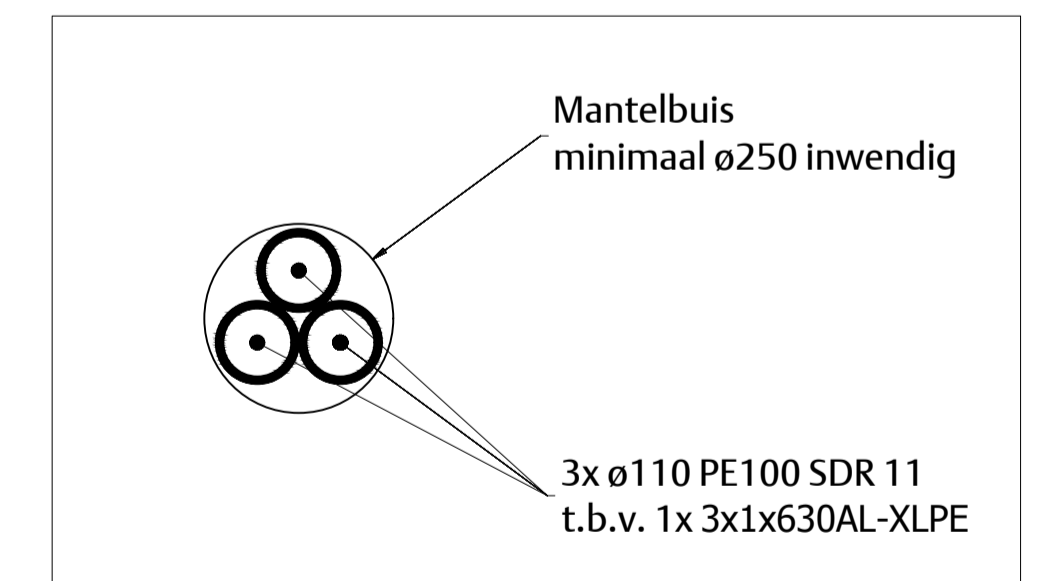
Doorsnede schaal 1 : 10
