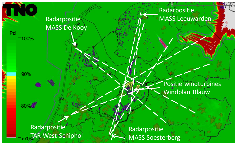
Figuur 12 Detectiekans van het primaire verkeersleidingsradarnetwerk berekend op 1000 voet in het schaduwgebied van het bouwplan nadat deze is gerealiseerd. Op dit figuur is detectiekansmiddeling toegepast. De stippellijnen geven aan waar de schaduw kan ontstaan.
