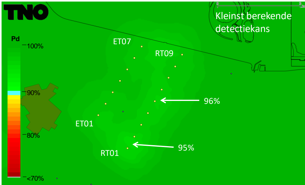
Figuur 10 Het gebied rond de windturbines Elandtocht (ET) en Rendiertocht (RT) uit Figuur 7 groter weergegeven.
