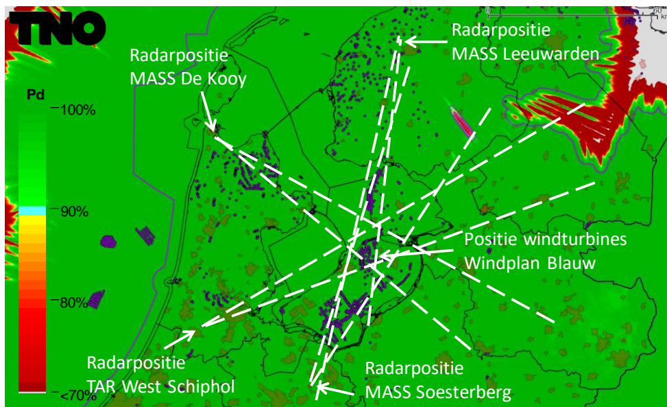
Figuur 11 Detectiekans van het primaire verkeersleidingsradarnetwerk op 1000 voet in het schaduwgebied van het bouwplan voordat deze is gerealiseerd (baseline). Op dit figuur is detectiekansmiddeling toegepast. De stippellijnen geven aan waar de schaduw kan gaan ontstaan.
