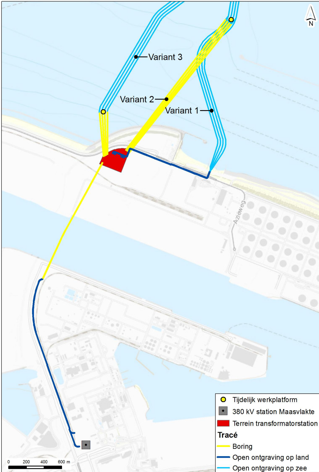
Afbeelding 2.1 Ligging drie aanlandingsvarianten
