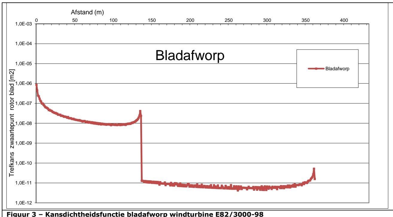
Figuur 3 – Kansdichtheidsfunctie bladafworp windturbine E82/3000-98
