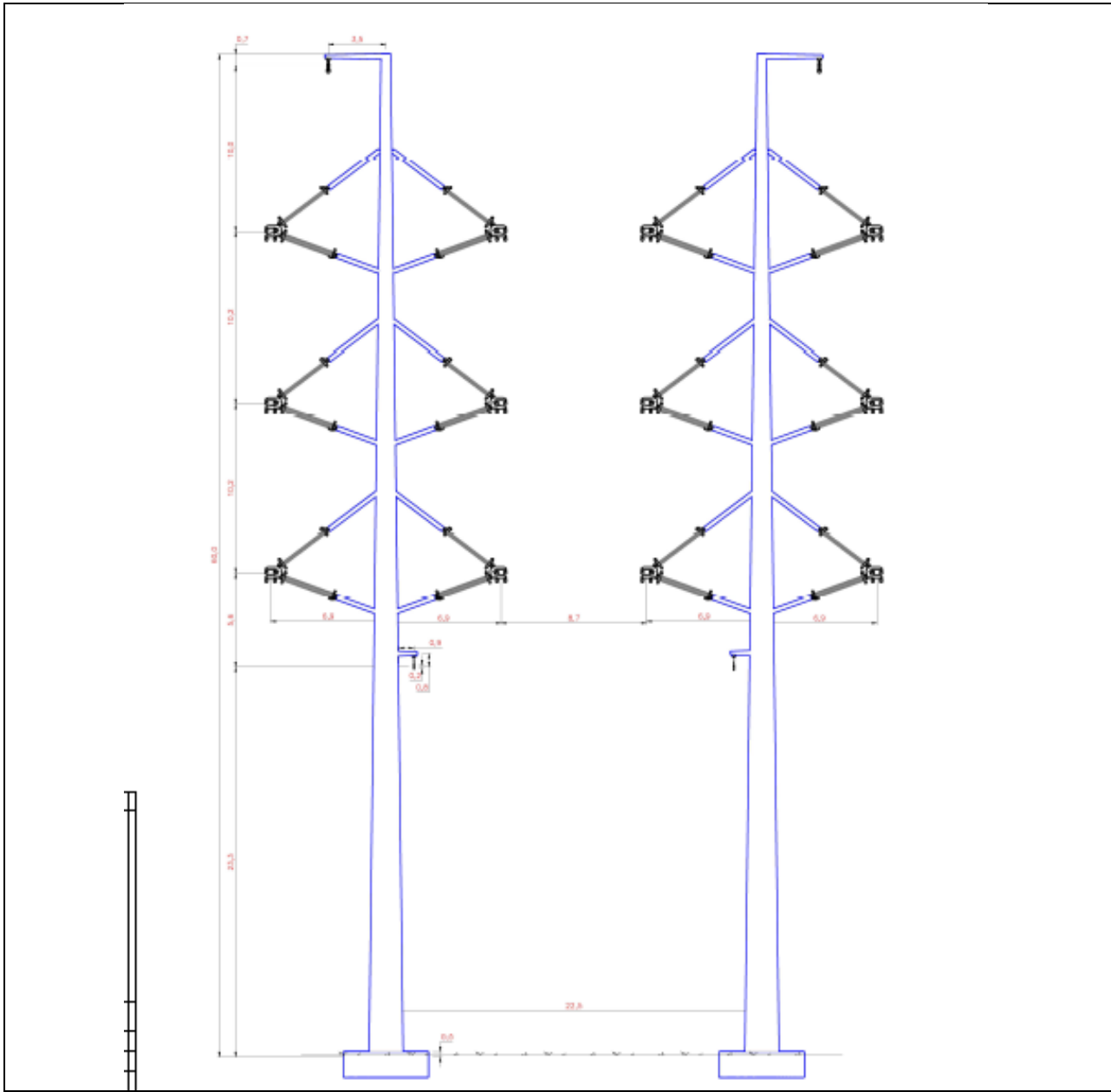
Figuur 2 – Wintrack viercircuit 380 kV steunmast (W6S400)
