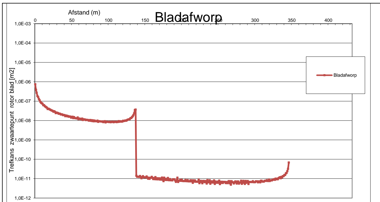
Figuur 4 – Kansdichtheidsfunctie bladafworp windturbine V112/3000-119
