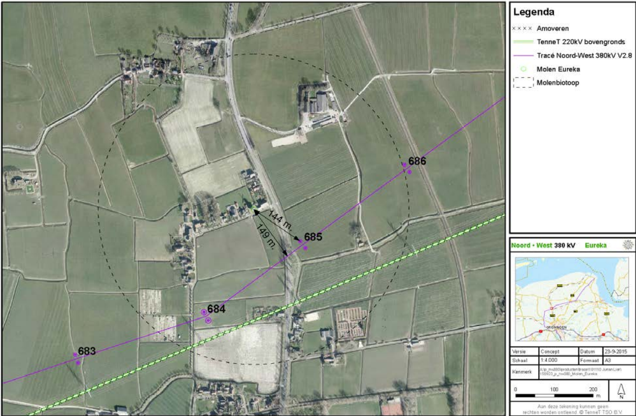
Figuur 4: Overzicht huidige en nieuwe situatie betreffende molen Eureka
