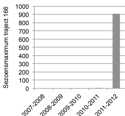
Figuur 4.22 Seizoenmaxima van toppers op open water op basis van de telgegevens van Rijkswaterstaat. Weergegeven zijn de maximum aantallen in traject 166 met bij-schattingen door RWS (zie kaart in bijlage 1 of figuur 3.2).
