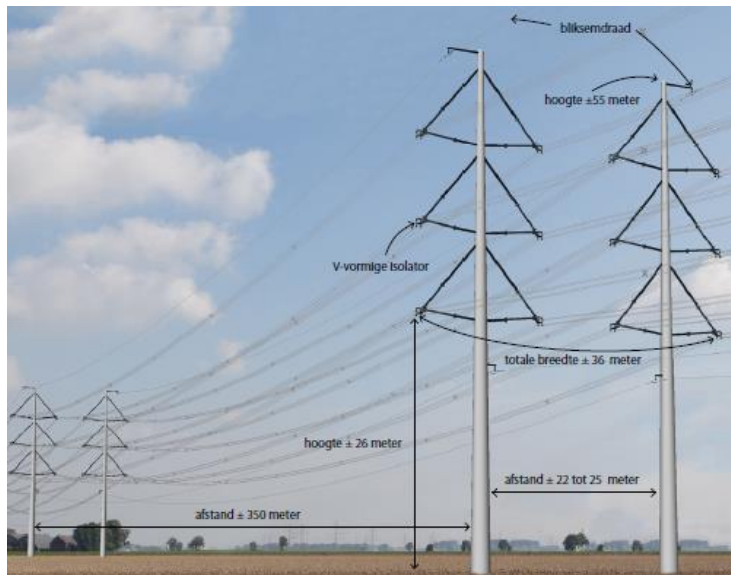
Afbeelding 2: Standaard Wintrackmast
