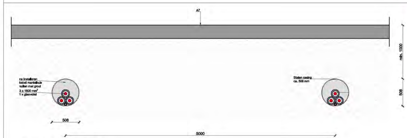
DOORSNEDE PERSBORING / RAKET BORING SCHAAL 1:20
