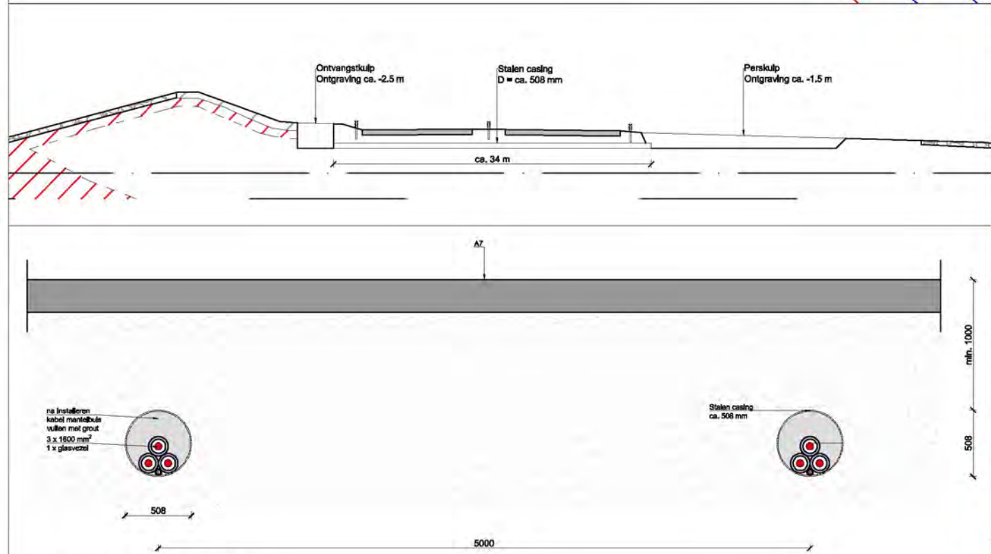
DOORSNEDE PERSBORING / RAKET BORING SCHAAL 1:20
