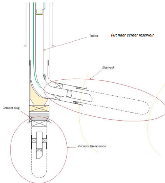
Figuur 3.2: Schematische afbeelding van een "sidetrack" boring
